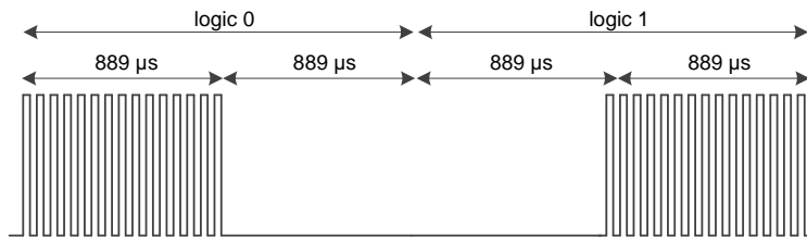
图 19. RC5 协议，位编码
