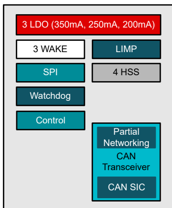
Figure 3-1. TCAN2855-Q1 Diagram
