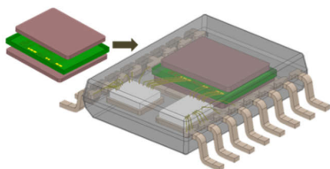
图 9. 磁耦合鐵氧體高性能變壓器。
