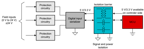
圖 13. PLC 數位輸入模組與隔離資料和功率。
