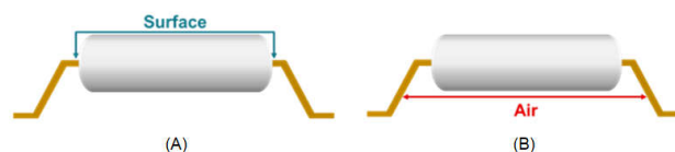
圖 3. 跨表面的爬電距離和通過隔離器封裝的空氣間隙。
