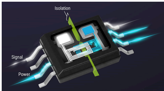
图 8. 使用磁隔離跨隔離層可靠地傳送電源和訊號。
