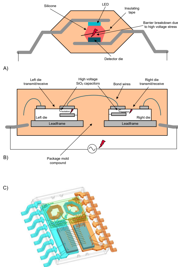
圖 4. 半導體隔離技術：光耦合器 (a)；電容式 (b)；變壓器 (c)。
