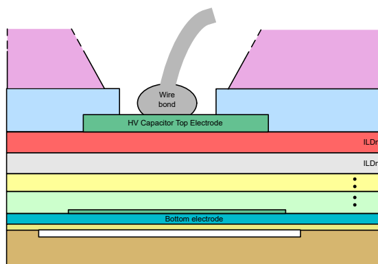
圖 7. Example cross-section of TI 的高壓隔離 SiO 2 電容器的截面積範例。
