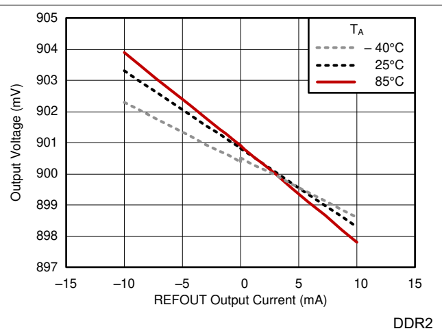
図 5-12. REFOUT 負荷レギュレーション
