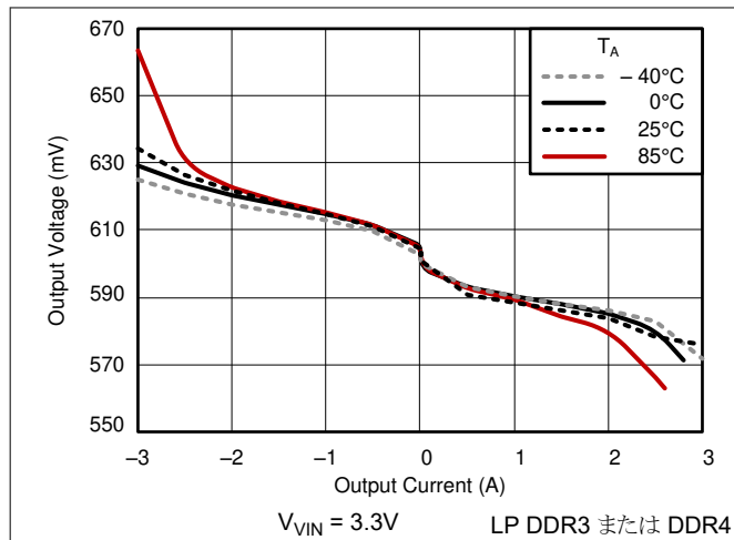
図 5-5. ロードレギュレーション
