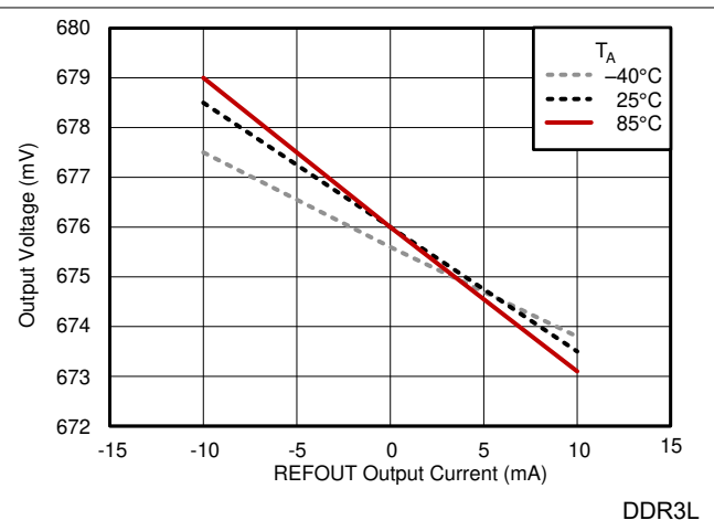
図 5-14. REFOUT 負荷レギュレーション
