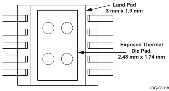
図 7-12. 推奨されるランドパッドパターン
