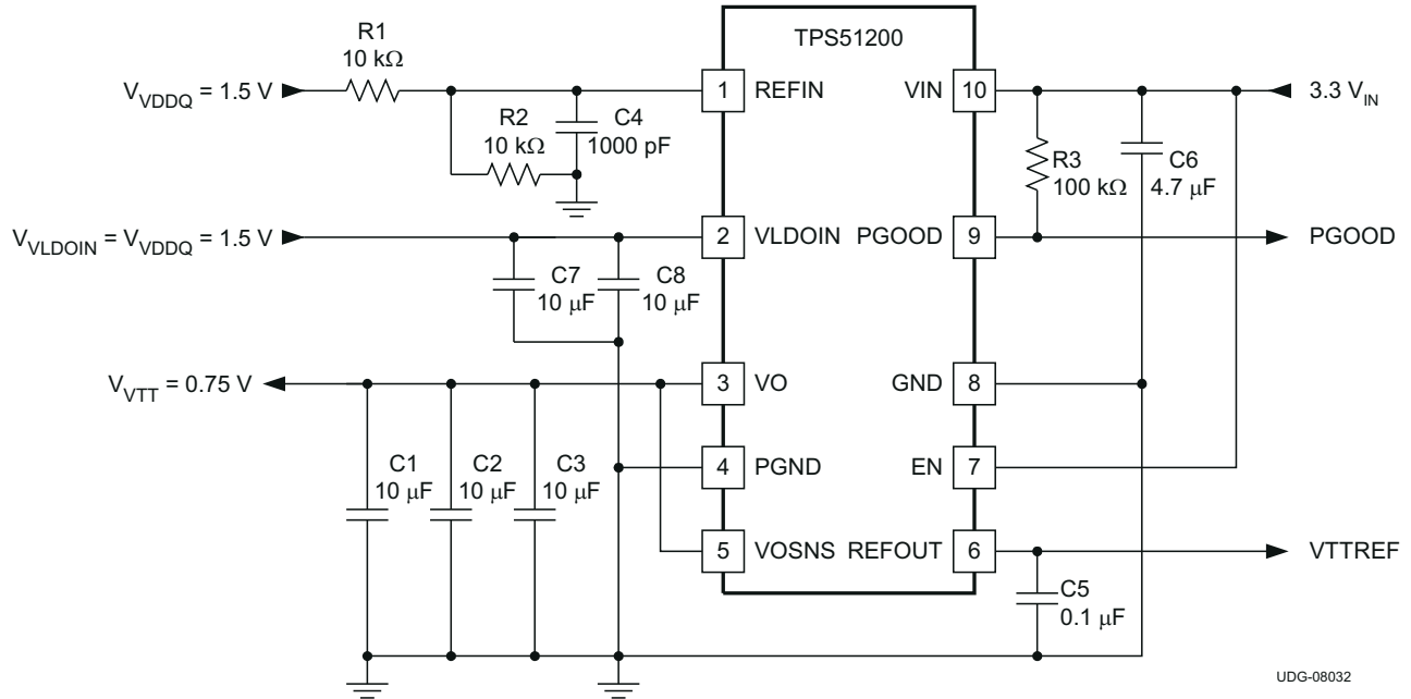
図 7-8. 3.3V IN 、DDR3 トラッキング構成
