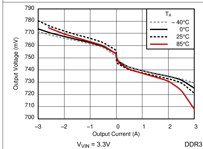
図 5-3. ロードレギュレーション
