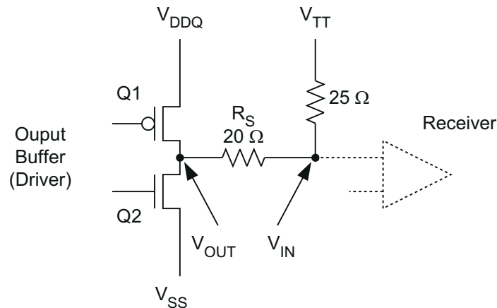
図 6-4. DDR 物理信号システム双方向 SSTL 信号伝達
