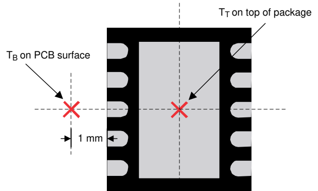
図 7-13. パッケージの熱測定
