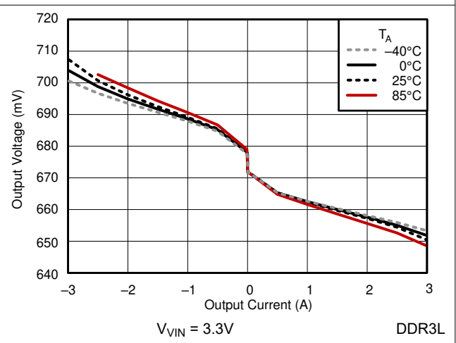
図 5-4. ロードレギュレーション
