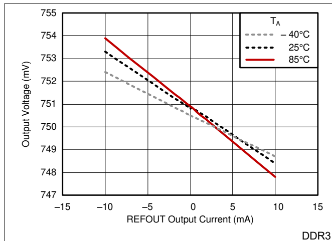
図 5-13. REFOUT 負荷レギュレーション
