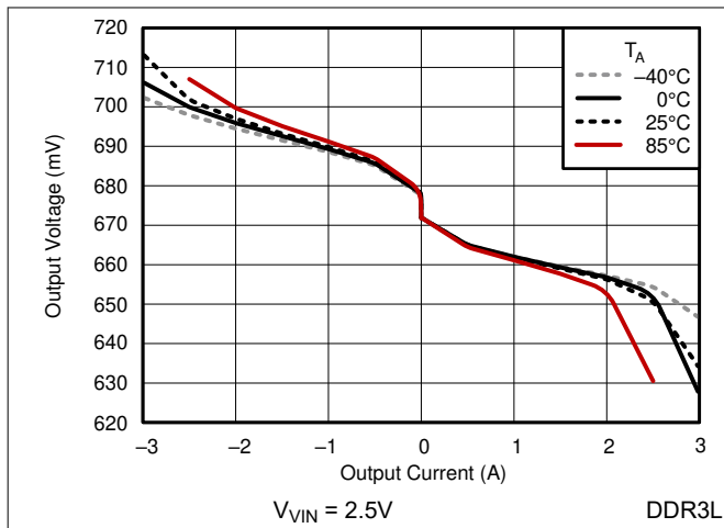
図 5-9. ロードレギュレーション
