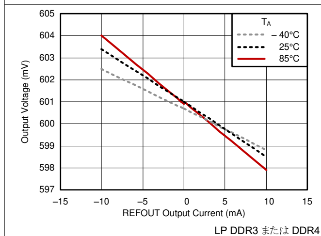
図 5-15. REFOUT 負荷レギュレーション
