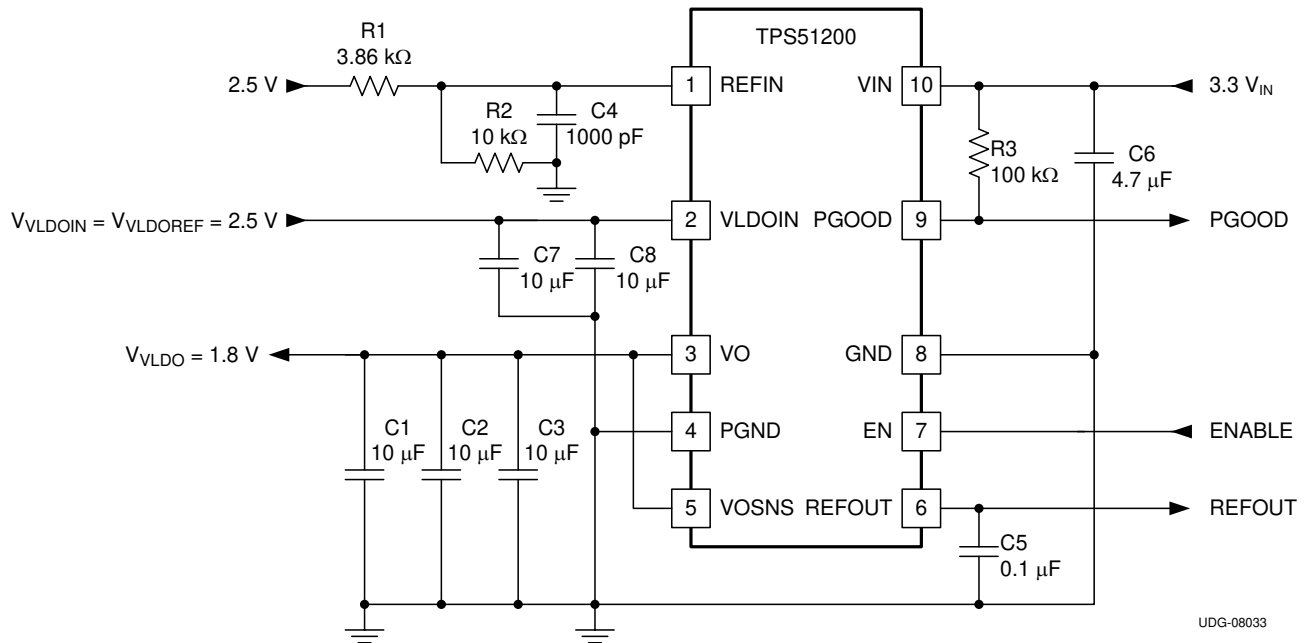
図 7-9. 3.3V IN LDO 構成
