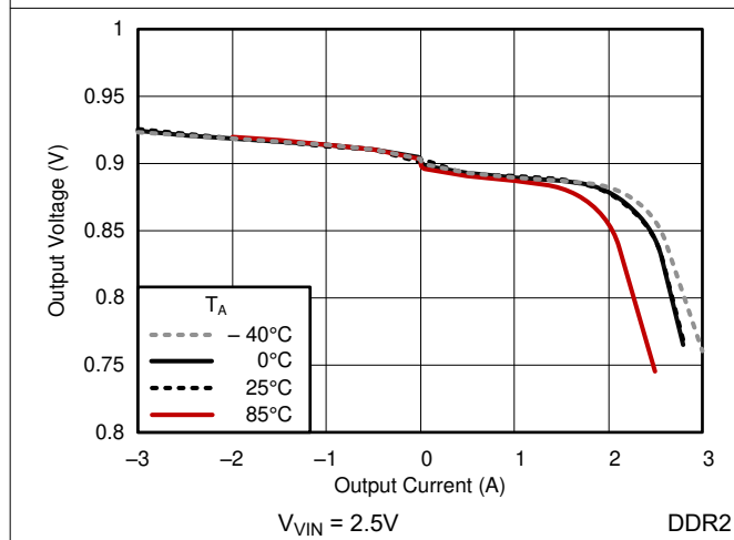
図 5-7. ロードレギュレーション
