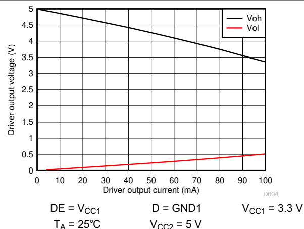
図 6-12. ドライバ出力電圧とドライバ出力電流との関係
