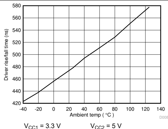
図 6-16. ISO141x ドライバの立ち上がり / 立ち下がり 時間 (ns) と温度 (°C) との関係
