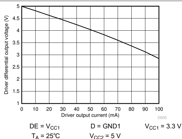
図 6-13. ドライバ差動出力電圧とドライバ出力電流との関係
