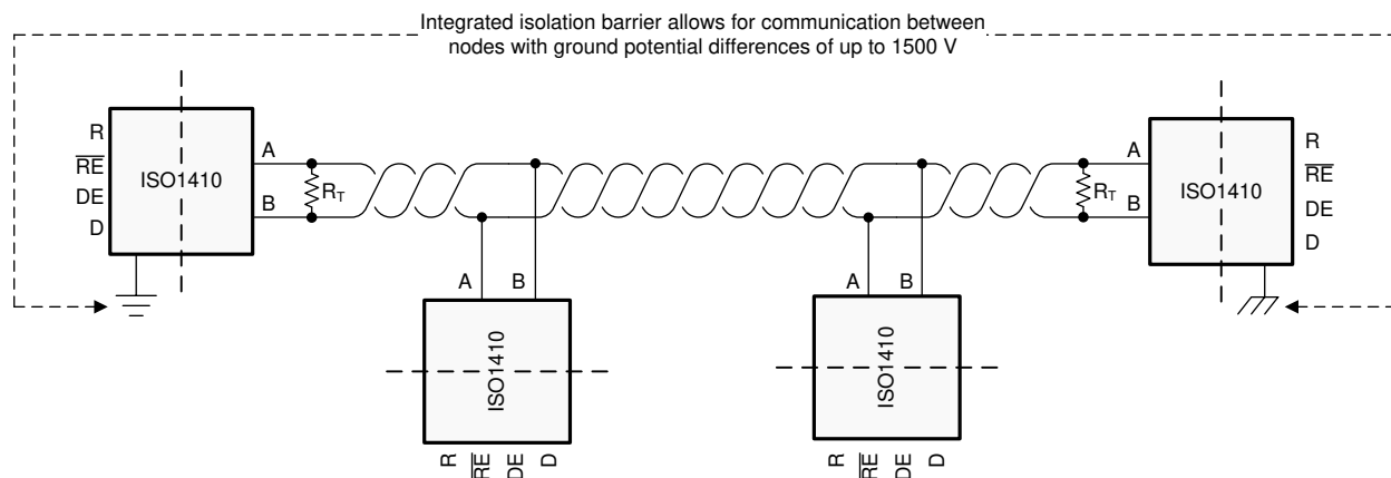
図 9-2. 半二重絶縁型トランシーバを使用した標準的な RS-485 ネットワーク
