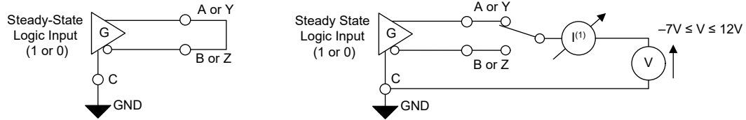
図 7-11. 短絡電流制限
