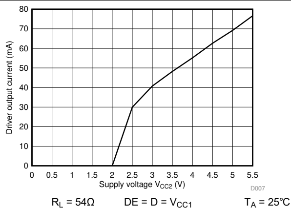
図 6-15. ドライバ出力電流と電源電圧との関係 ( V_{CC2} )
