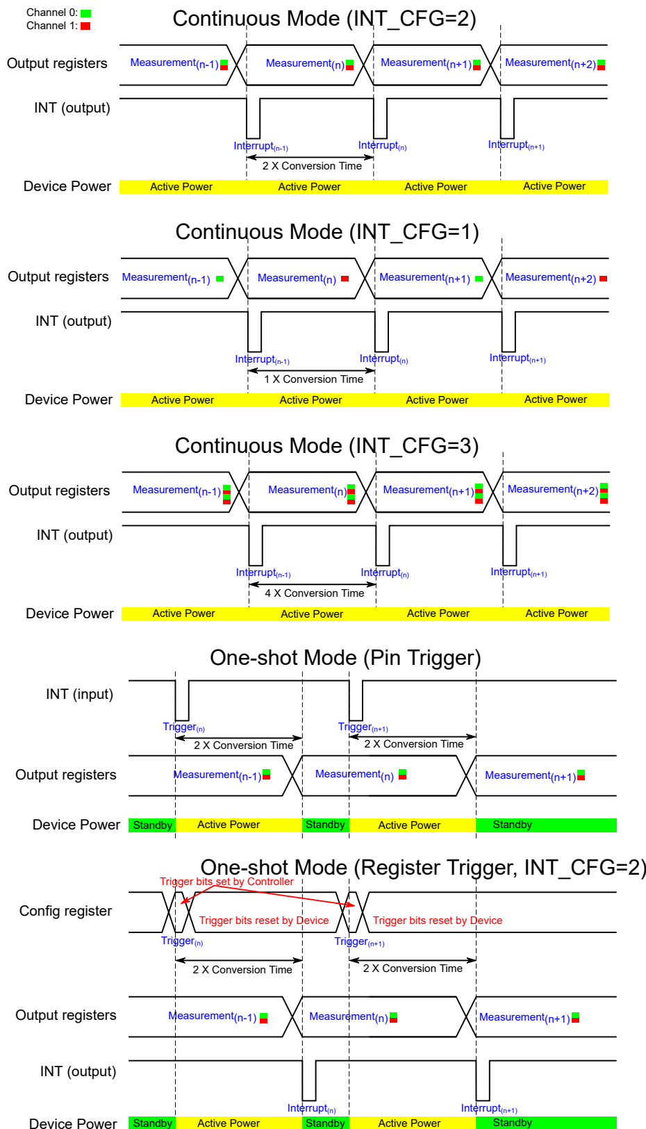
図 6-2. 各種動作モードのタイミング図
