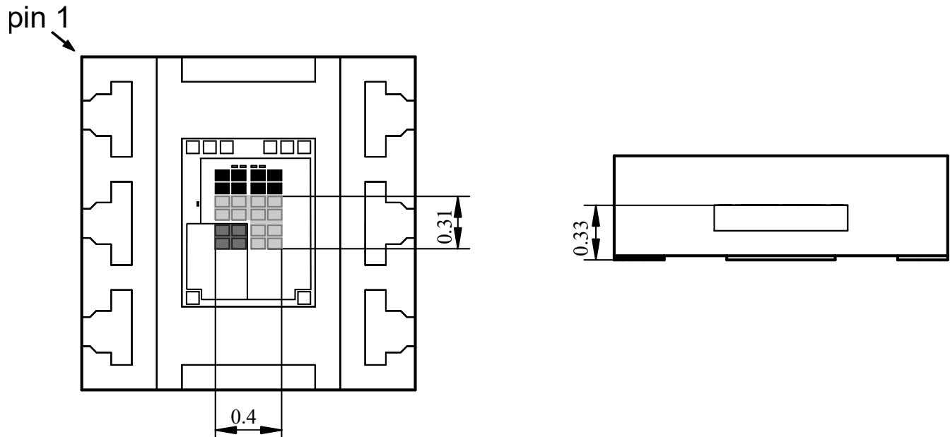
図 8-2. USON センサの位置
