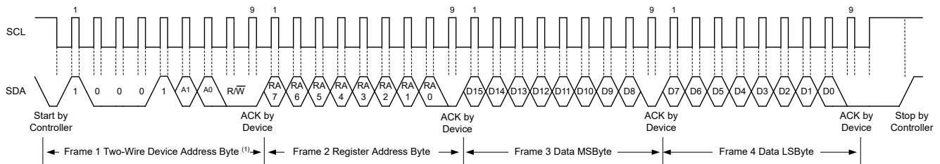
図 6-5. I 2 C 書き込み例
