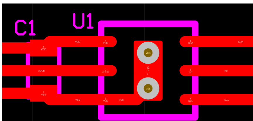
図 8-6. DNP パッケージのレイアウト例
