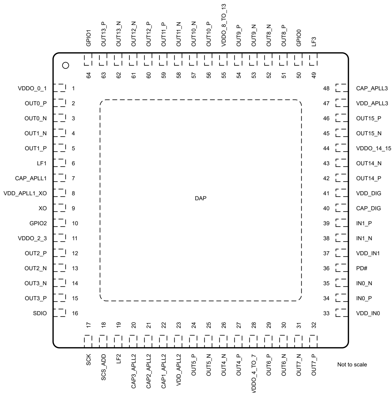
図 5-1. LMK5B33216 RGC パッケージ、64 ピン VQFN 上面図
