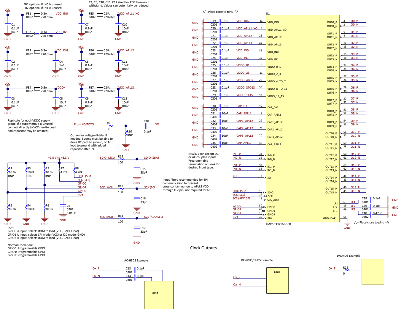
図 9-4. 代表的なアプリケーションの例
