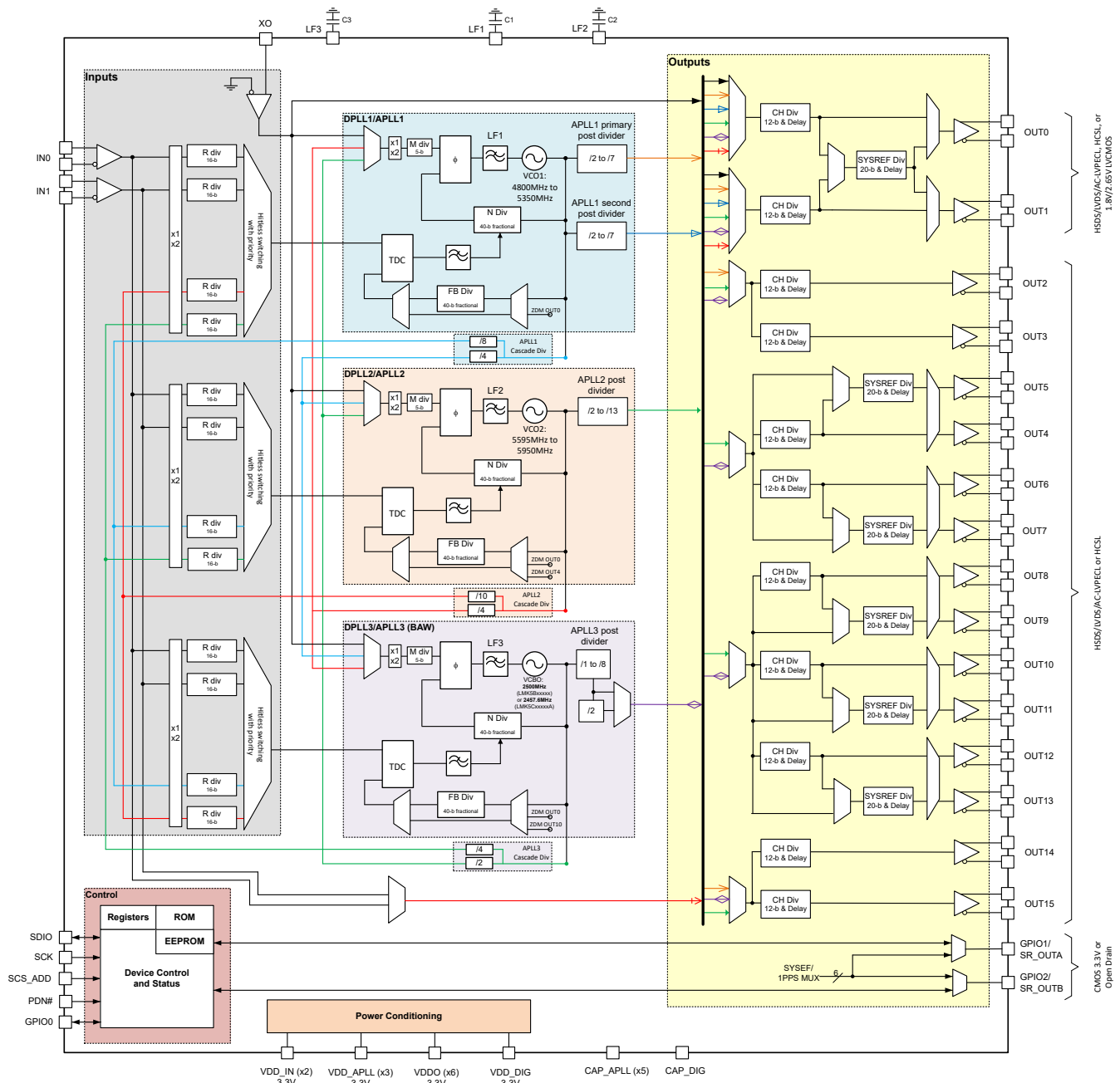
図 8-1. LMK5B33216 最上位ブロック図
