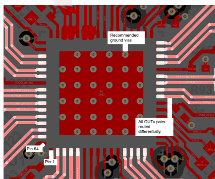
図 9-6. LMK5B33216 の PCB レイアウト例、最上層
