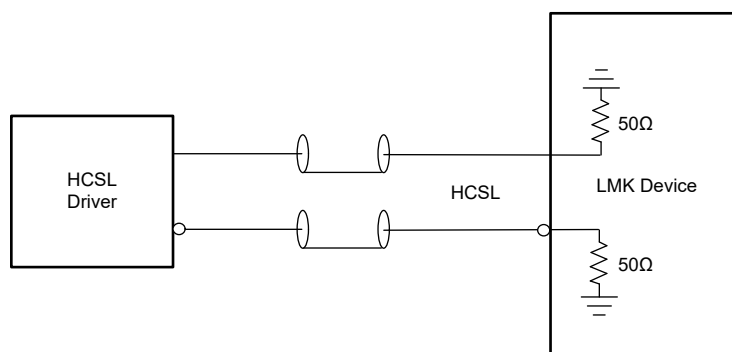
図 8-14. HCSL (負荷終端) からレファレンス (INx)
