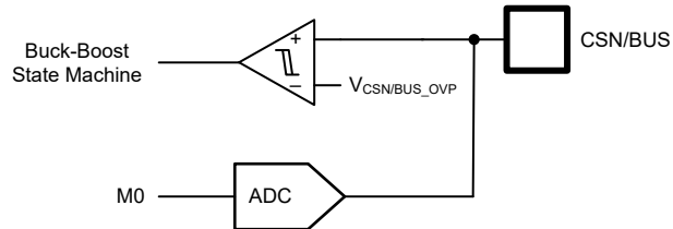
図 8-17. V_{BUS} OVP と UVP
