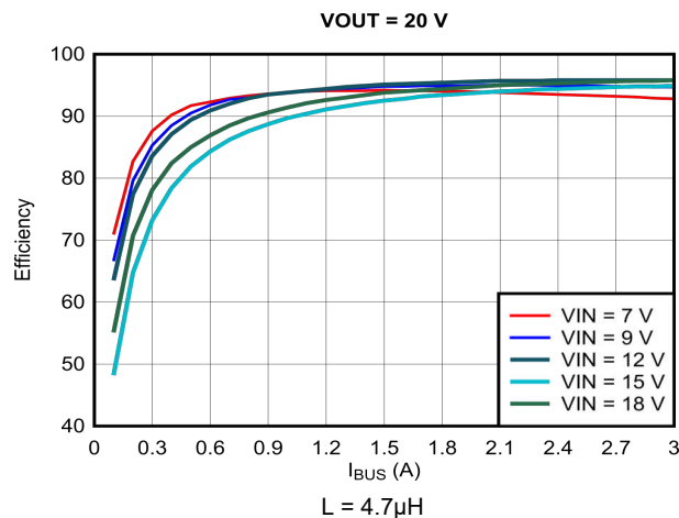
図 9-10. 効率と出力電流 ( I_{OUT} )、 V_{OUT} = 20V との関係
