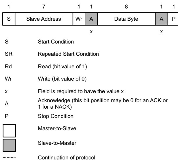
図 8-40. I 2 C 読み取り / 書き込みのプロトコル キー
