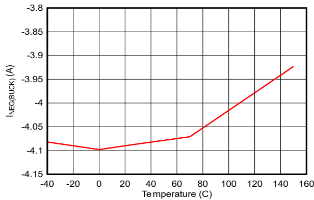
図 6-21. 降圧負電流制限と温度との関係
