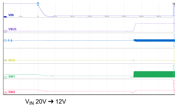
図 9-28. V IN(OVP) 回復
