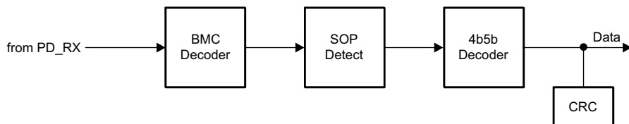
図 8-20. USB-PD ベースバンド レシーバのブロック図
