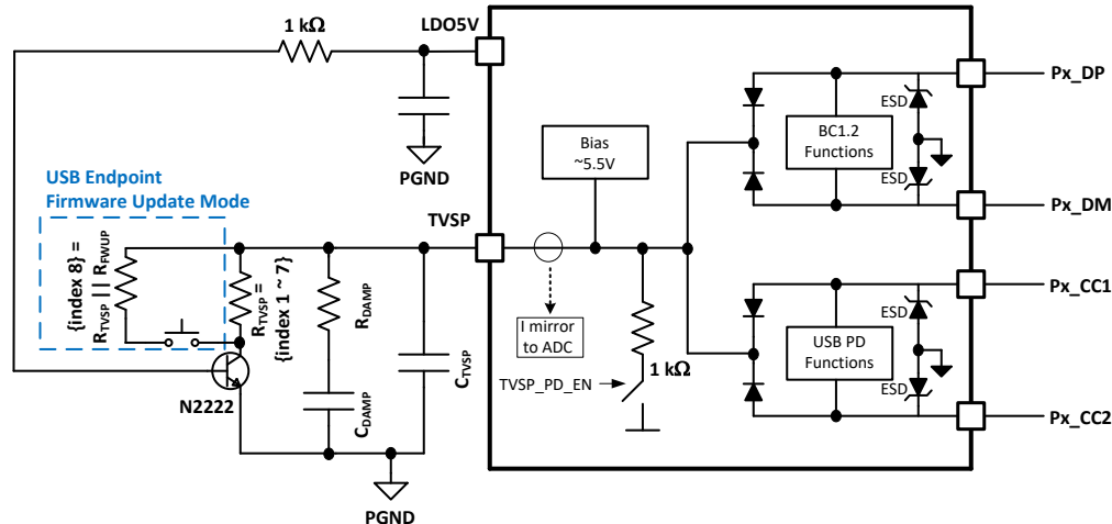
図 8-6. USB エンドポイントのファームウェア アップデート モードを有効にする回路の例
