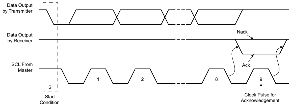
図 8-37. I 2 C 応答確認
