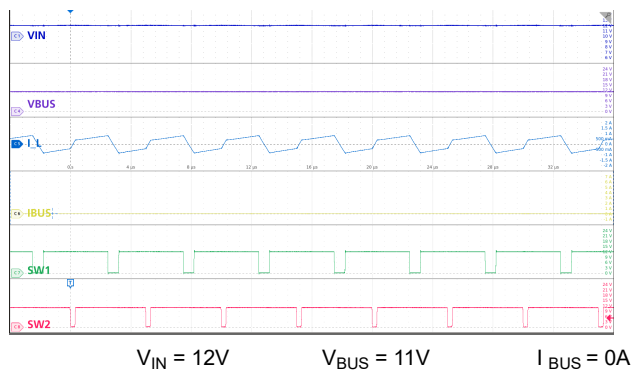
図 9-23. 昇降圧モード : V_{IN} \neq V_{BUS} 、無負荷
