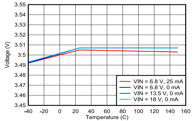
図 6-10. LDO_3V3、 V_{IN} と温度との関係
