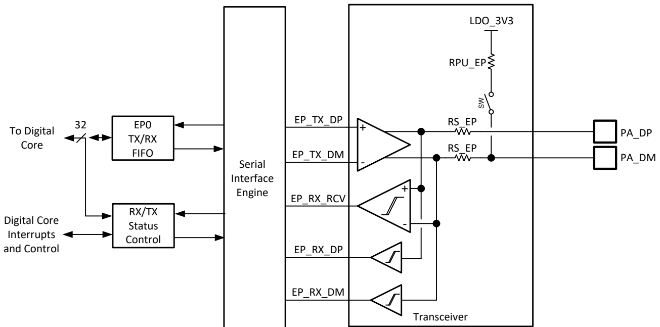
図 8-33. USB エンドポイント PHY
