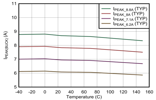
図 6-20. 降圧ピーク電流制限と温度との関係 (低設定)
