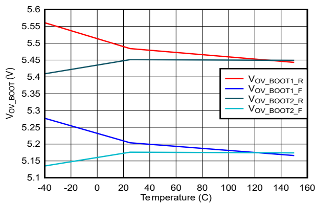
図 6-23. BOOTx OVP と温度との関係
