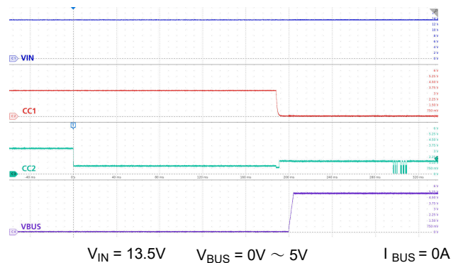
図 9-12. Type-C 接続
