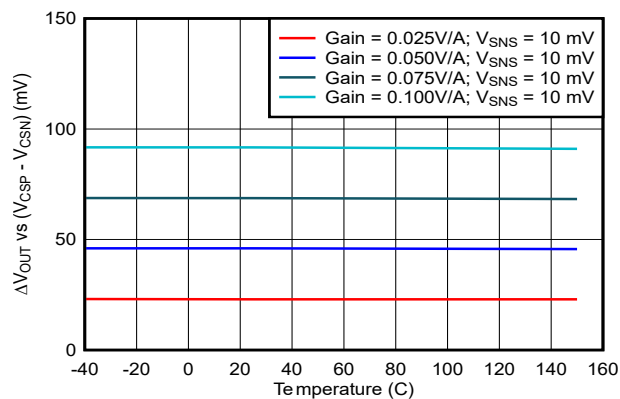
図 6-29. ケーブル電圧ドロップ補償と温度との関係
