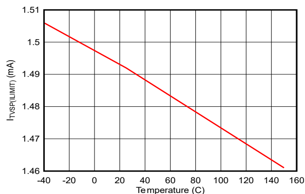
図 6-15. I_{TVSP(ILIMIT)} と温度との関係
