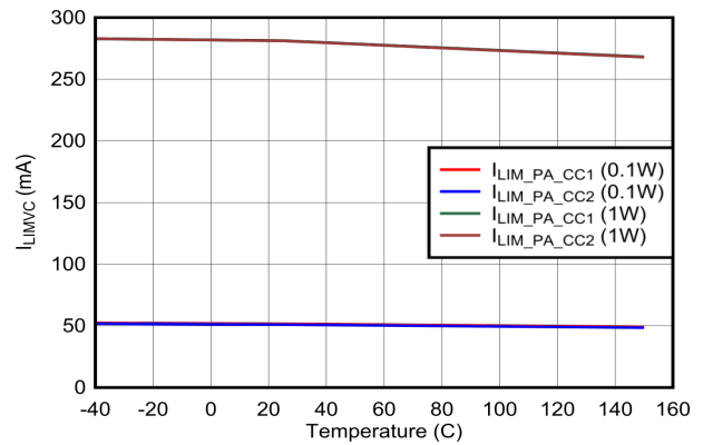
図 6-40. V_{CONN} パワーパス : 電流制限と温度との関係
