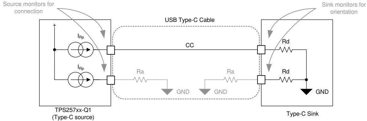
図 8-28. Type-C ケーブル
