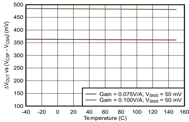
図 6-31. ケーブル電圧ドロップ補償と温度との関係
