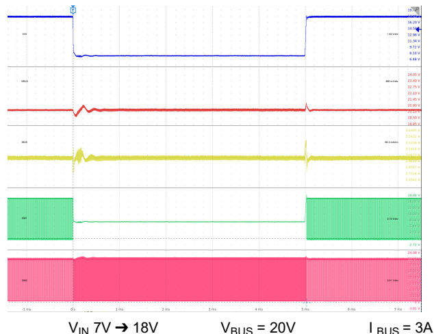
図 9-35. ライン過渡： V_{BUS} = 20V
