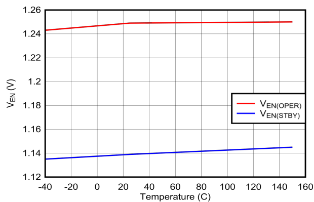
図 6-3. ENABLE/UVLO スレッシュホールドと温度との関係
