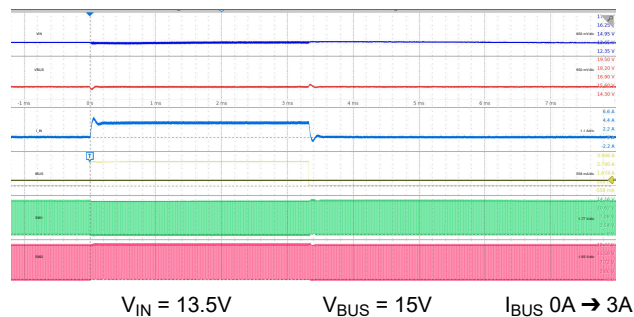
図 9-32. 負荷過渡 (昇降圧) : V BUS = 15V
