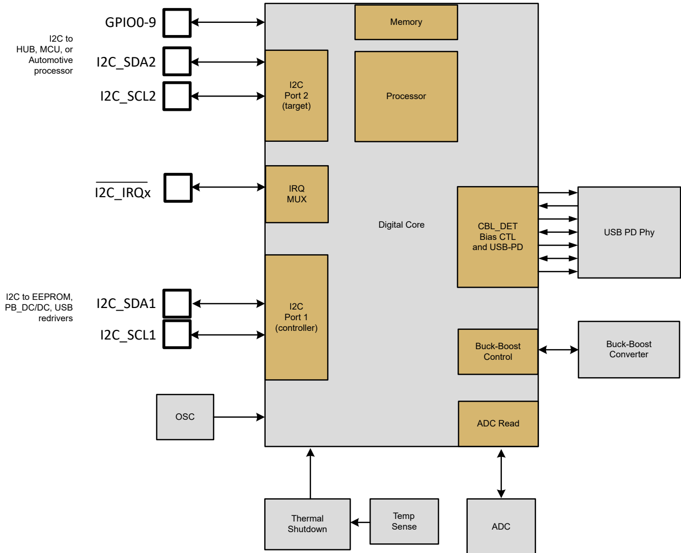
図 8-41. デジタル コアの簡略化されたブロック図
