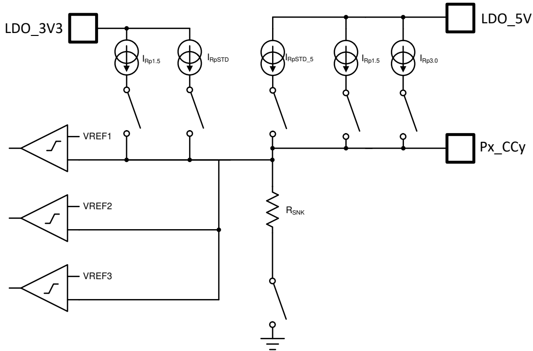
図 8-27. プラグおよび方向検出ブロック
