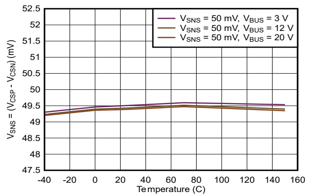
電流制限時の目標 V_{SNS} = 50mV 電流制限作動
