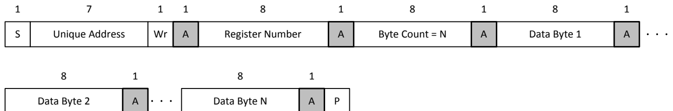
図 8-38. I 2 C 固有アドレス書き込みレジスタ プロトコル
