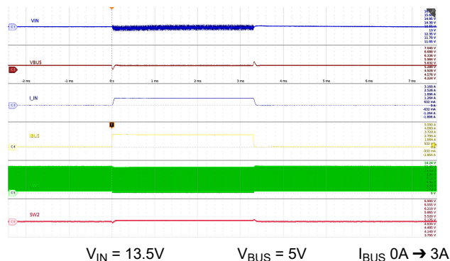
図 9-30. 負荷過渡 (降圧) : V BUS = 5V
