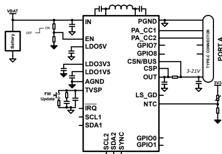
図 9-1. 簡易シングル USB PD チャージャ
