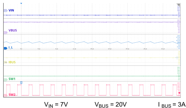
図 9-16. 昇圧モード：低 V_{IN} 、3A 負荷
