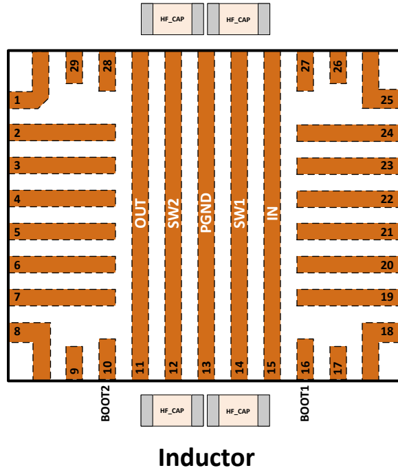
図 9-4. 入力および出力 C_{HF} コンデンサの配置
