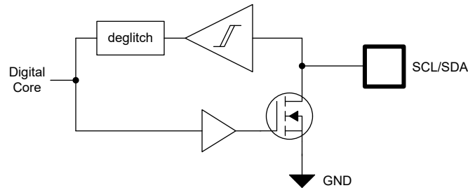
図 8-34. I 2 C ドライバ
