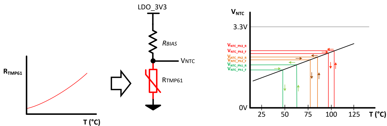
図 8-44. TMP61 の PTC 応答曲線
