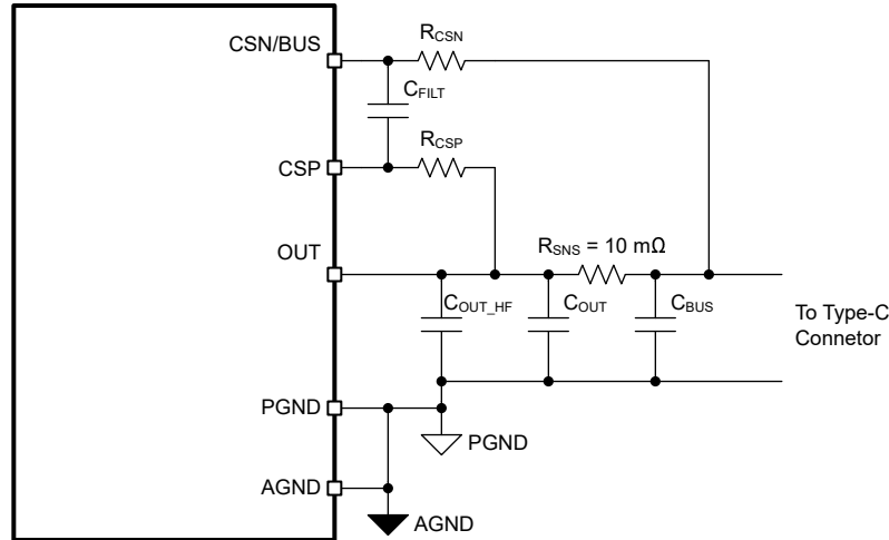
図 9-5. 電流センス アンプ : RC フィルタ部品
