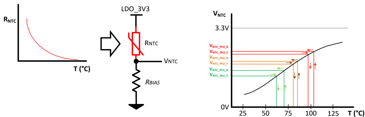
図 8-43. NTC 応答曲線
