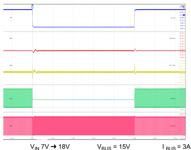
図 9-36. ライン過渡： V_{BUS} = 15V
