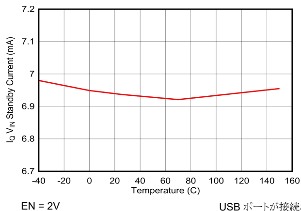
図 6-2. I_Q V_{IN} のスタンバイ電流の温度特性
