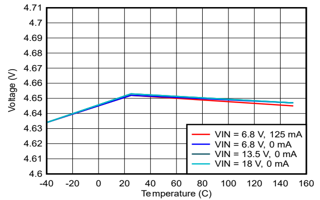
図 6-8. LDO_5V、 V_{IN} と温度との関係
