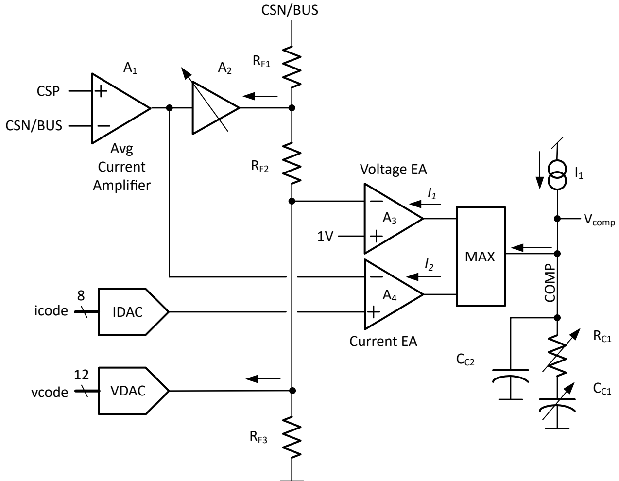
図 8-16. フィードバックパスとエラーアンプの簡略ブロック図。
