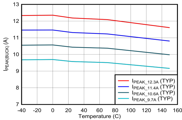
図 6-19. 降圧ピーク電流制限と温度との関係 (高設定)
