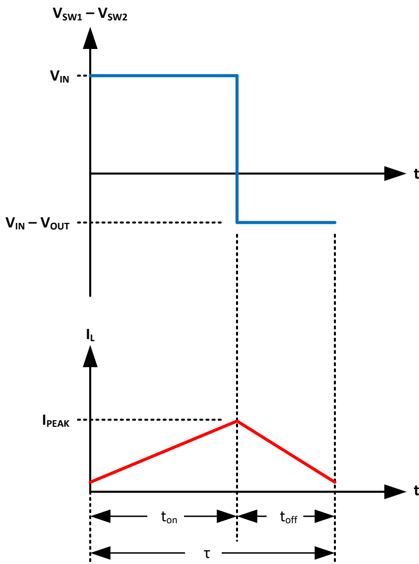
図 8-11. 昇圧状態
