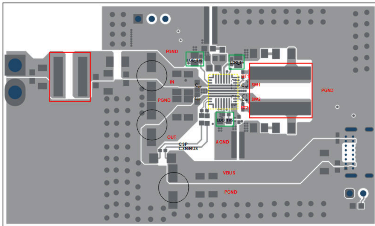
図 9-39. TPS25762-Q1 電力段のレイアウト
