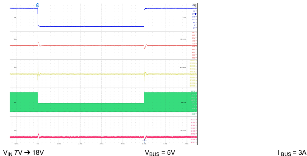
図 9-38. ライン過渡： V_{BUS} = 5V
