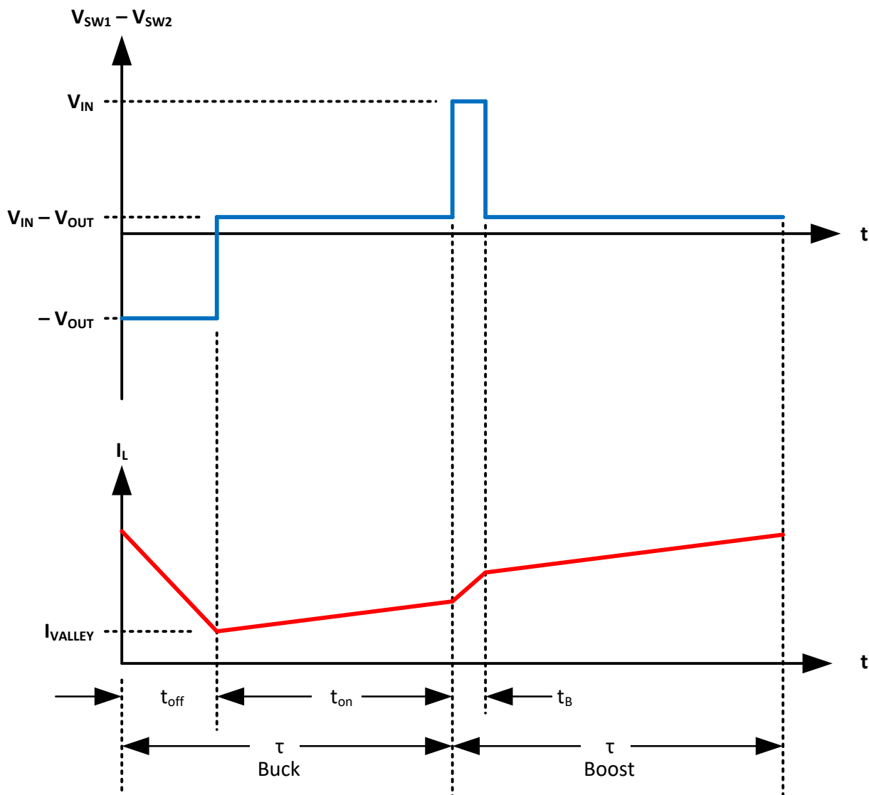
図 8-9. 降圧遷移
