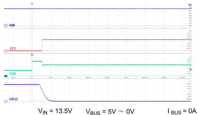
図 9-13. Type-C 接続解除
