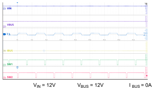
図 9-22. 昇降圧モード : V_{IN} = V_{BUS} 、無負荷
