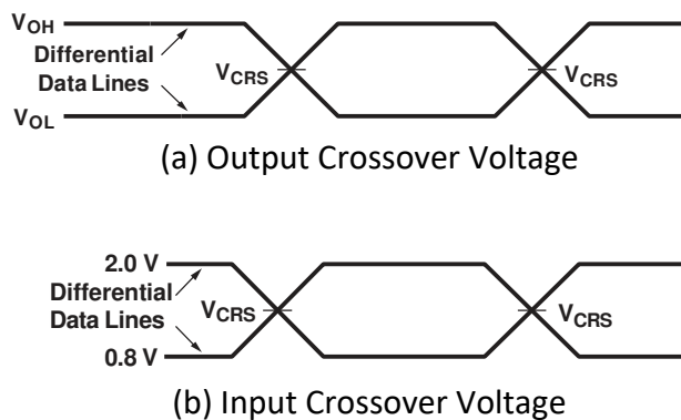
図 7-4. USB エンドポイントのクロスオーバー電圧
