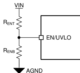
図 8-2. UVLO スレッショルドのプログラミング
