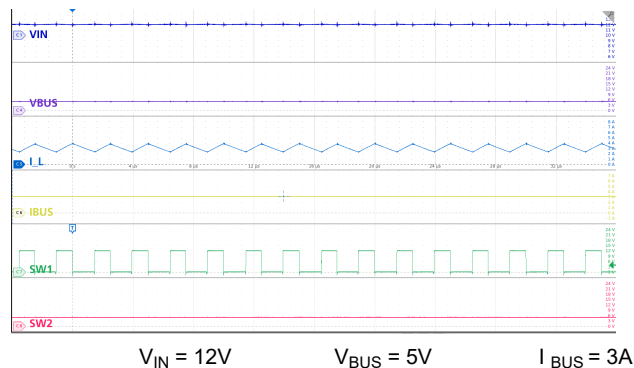
図 9-20. 降圧モード：公称 V_{IN} 、3A 負荷
