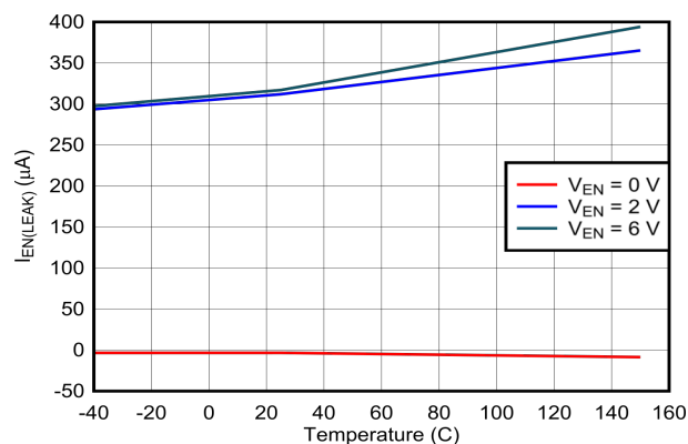
図 6-5. EN リーク電流と温度との関係
