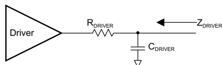
図 8-24. ZDRIVER 回路
