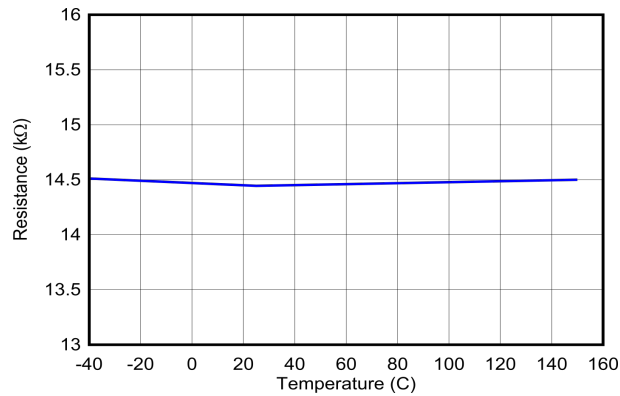
図 6-43. USB BC1.2 : DM から AGND への 15kΩ 抵抗、 R_{DM\_DWN\_15k}
