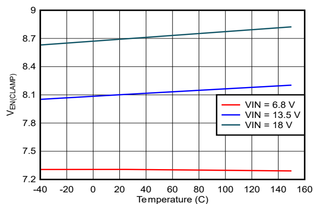
図 6-4. EN クランプ電圧と温度との関係
