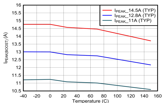
図 6-17. 昇圧ピーク電流制限と温度との関係 (高設定)
