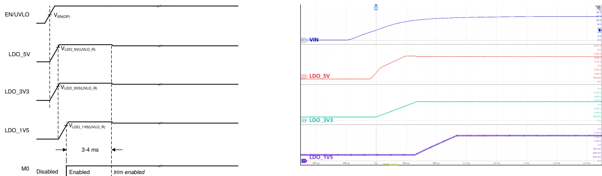
図 8-1. EN/UVLO と LDO のシーケンシング
