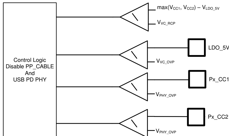
図 8-29. 過電圧および逆電流保護
