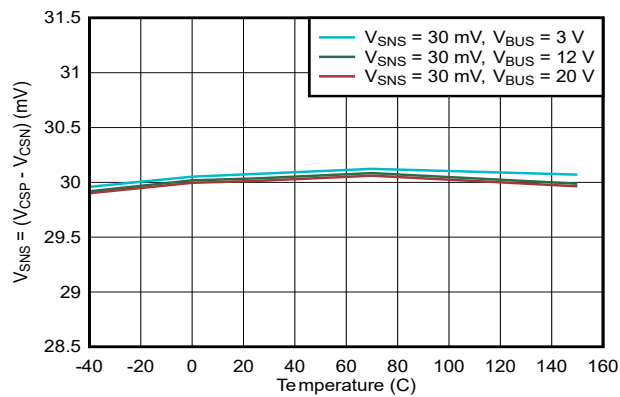
電流制限時の目標 V_{SNS} = 30mV 電流制限作動
