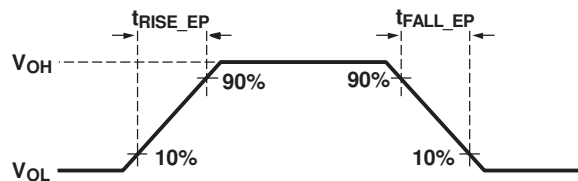
図 7-3. USB エンドポイント トランスミッタの立ち上がり時間および立ち下がり時間
