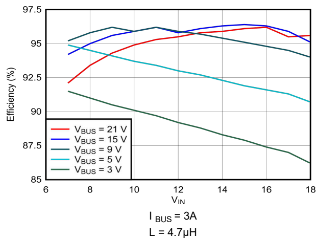
図 9-11. 効率と入力電圧との関係
