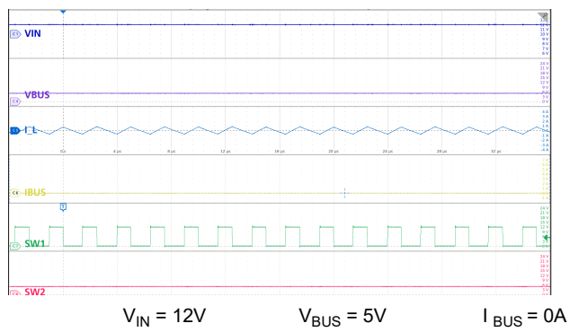
図 9-19. 降圧モード：公称 V_{IN} 、無負荷
