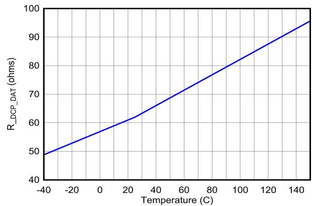
図 6-42. USB BC1.2 : DP から DM への短絡抵抗、 R_{DCP\_DAT}
