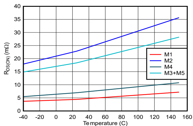
図 6-16. 昇降圧パワー FET の R_{DS(ON)} と温度との関係
