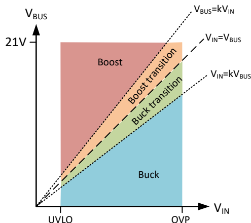
図 8-12. 動作領域
