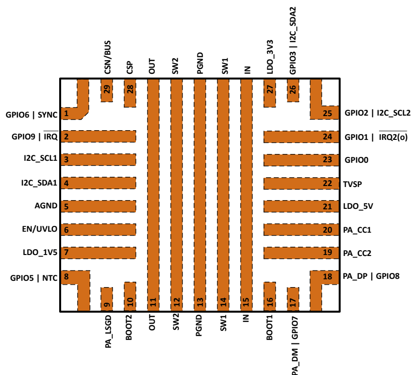
図 5-1. TPS25762-Q1 RQL パッケージ、29 ピン VQFN (上面図)
