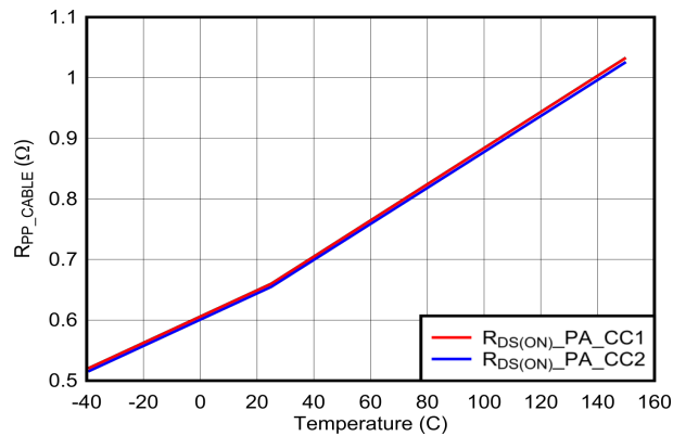
図 6-39. V_{CONN} パワーパス : R_{DS(ON)} と温度との関係
