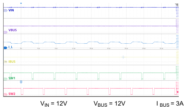
図 9-24. 昇降圧モード : V_{IN} = V_{BUS} 、3A 負荷
