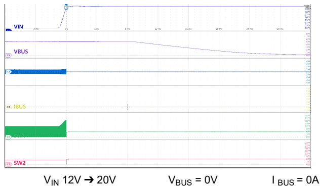
図 9-29. V IN(OVP) 時の V BUS 放電
