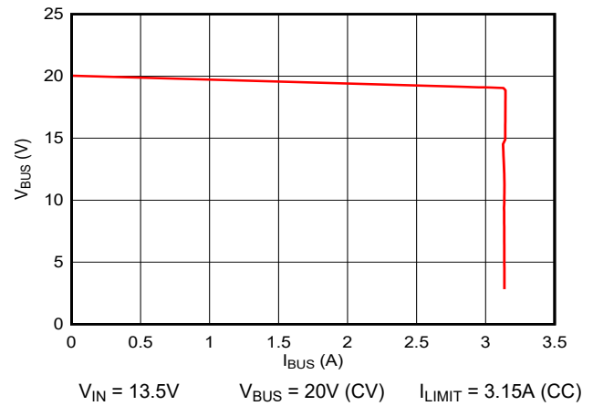
図 6-32. 定電圧から定電流への遷移
