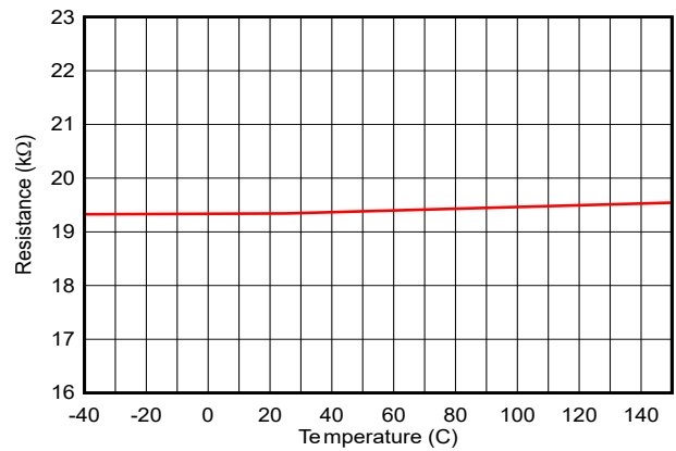
図 6-44. USB BC1.2 : DM から AGND への 20kΩ 抵抗、 R_{DM\_DWN\_20k}
