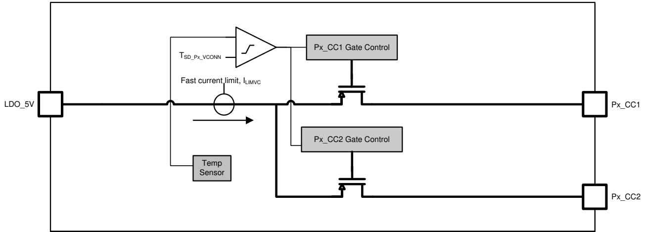
図 8-26. VCONN パワー スイッチ
