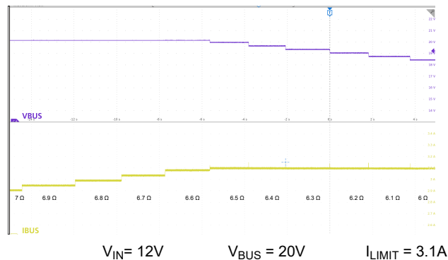
図 9-34. 電流制限：ステップ型抵抗性負荷
