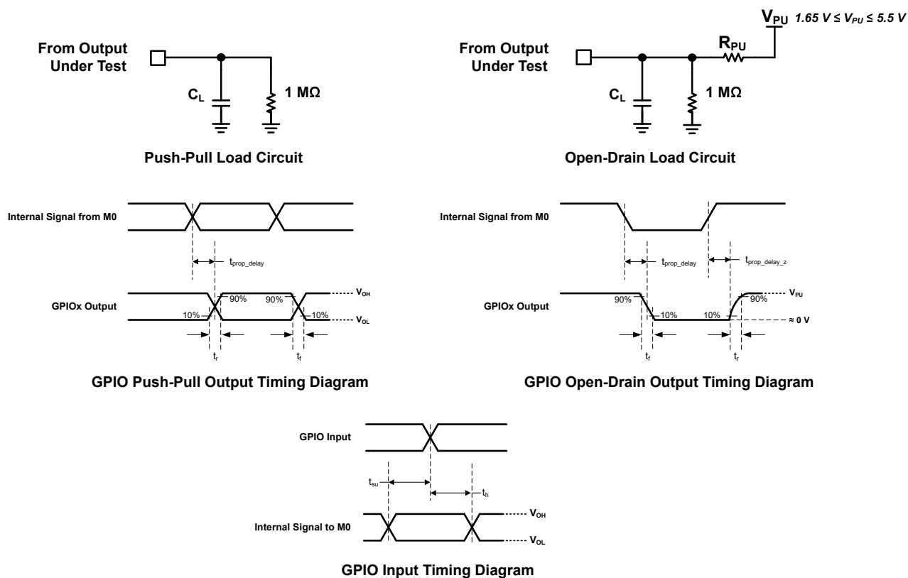
図 7-2. GPIO 出力のタイミング図 (立ち上がり / 立ち下がり と容量性負荷との関係)
