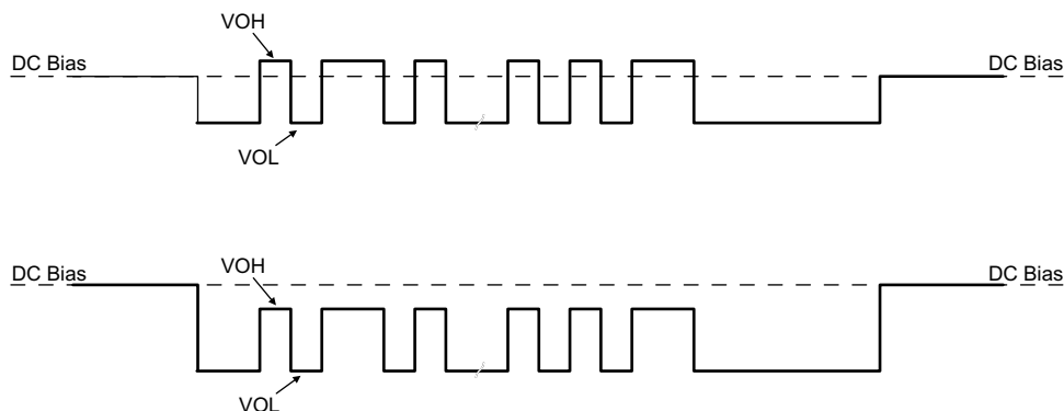
図 8-23. DC バイアスでの TX ドライバの送信
