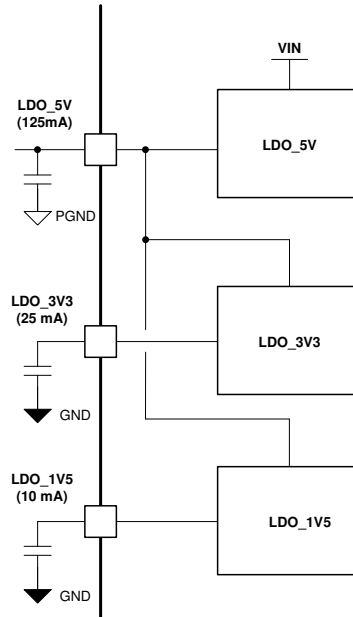
図 8-3. 内部 LDO のピン配置
