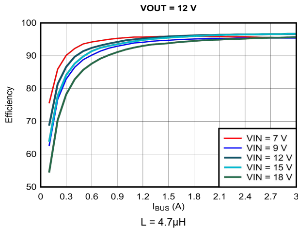
図 9-8. 効率と出力電流 ( I_{OUT} )、 V_{OUT} = 12V との関係
