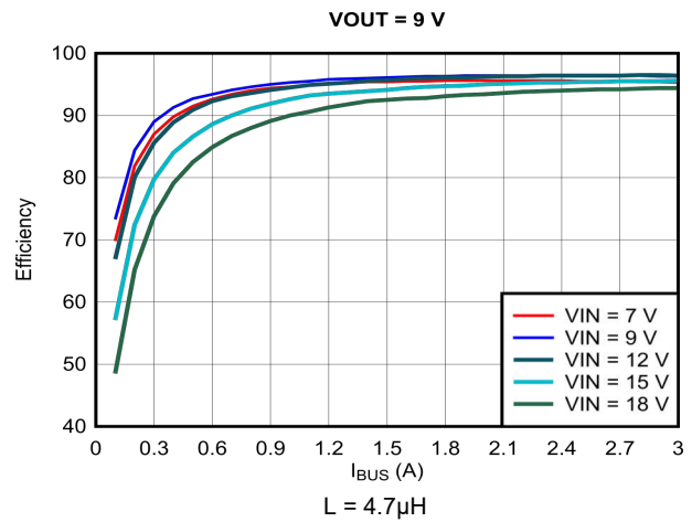
図 9-7. 効率と出力電流 ( I_{OUT} )、 V_{OUT} = 9V との関係
