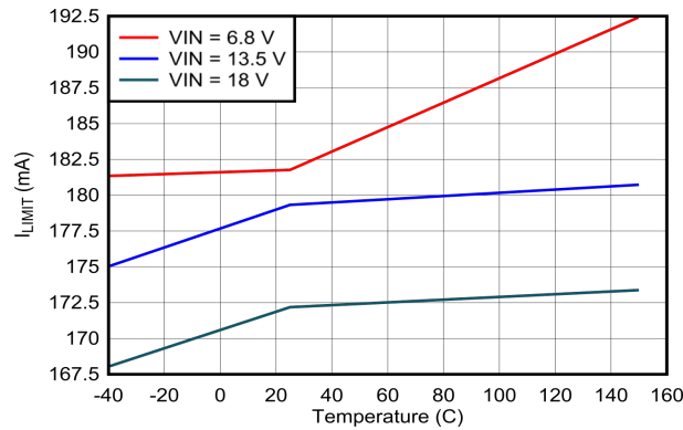
図 6-9. LDO_5V 電流制限、 V_{IN} と温度との関係
