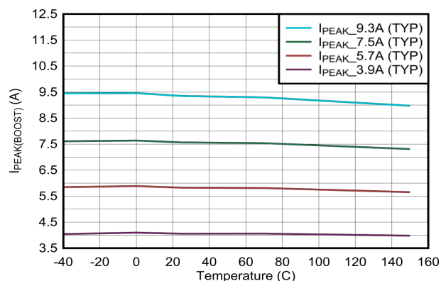
図 6-18. 昇圧ピーク電流制限と温度との関係 (低設定)
