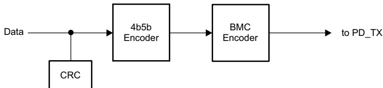
図 8-19. USB-PD ベースバンド トランスミッタのブロック図
