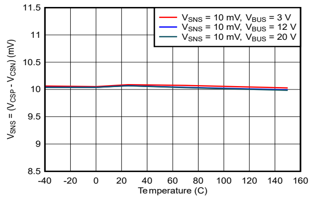
電流制限時の目標 V_{SNS} = 10mV 電流制限作動
