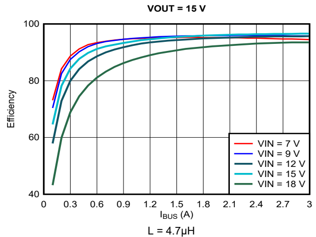
図 9-9. 効率と出力電流 ( I_{OUT} )、 V_{OUT} = 15V との関係
