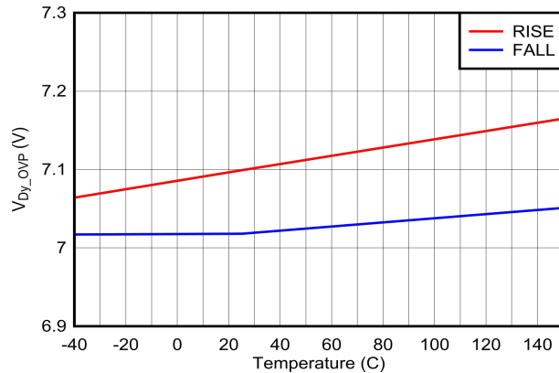
図 6-45. USB BC1.2: DP および DM ピンの過電圧保護スレッシュホールドと温度との関係
