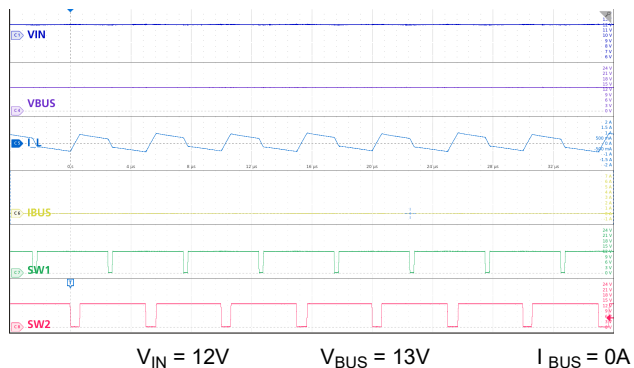
図 9-21. 昇降圧モード： V_{IN} \neq V_{BUS} 、無負荷
