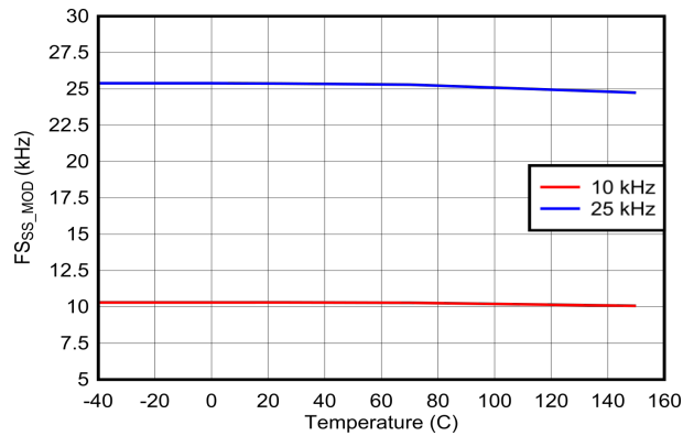
図 6-25. f_{sw} デザイン変調周波数と温度との関係
