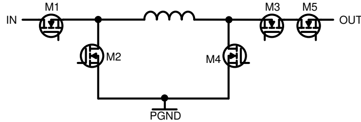
図 8-7. 昇降圧内部パワー FET
