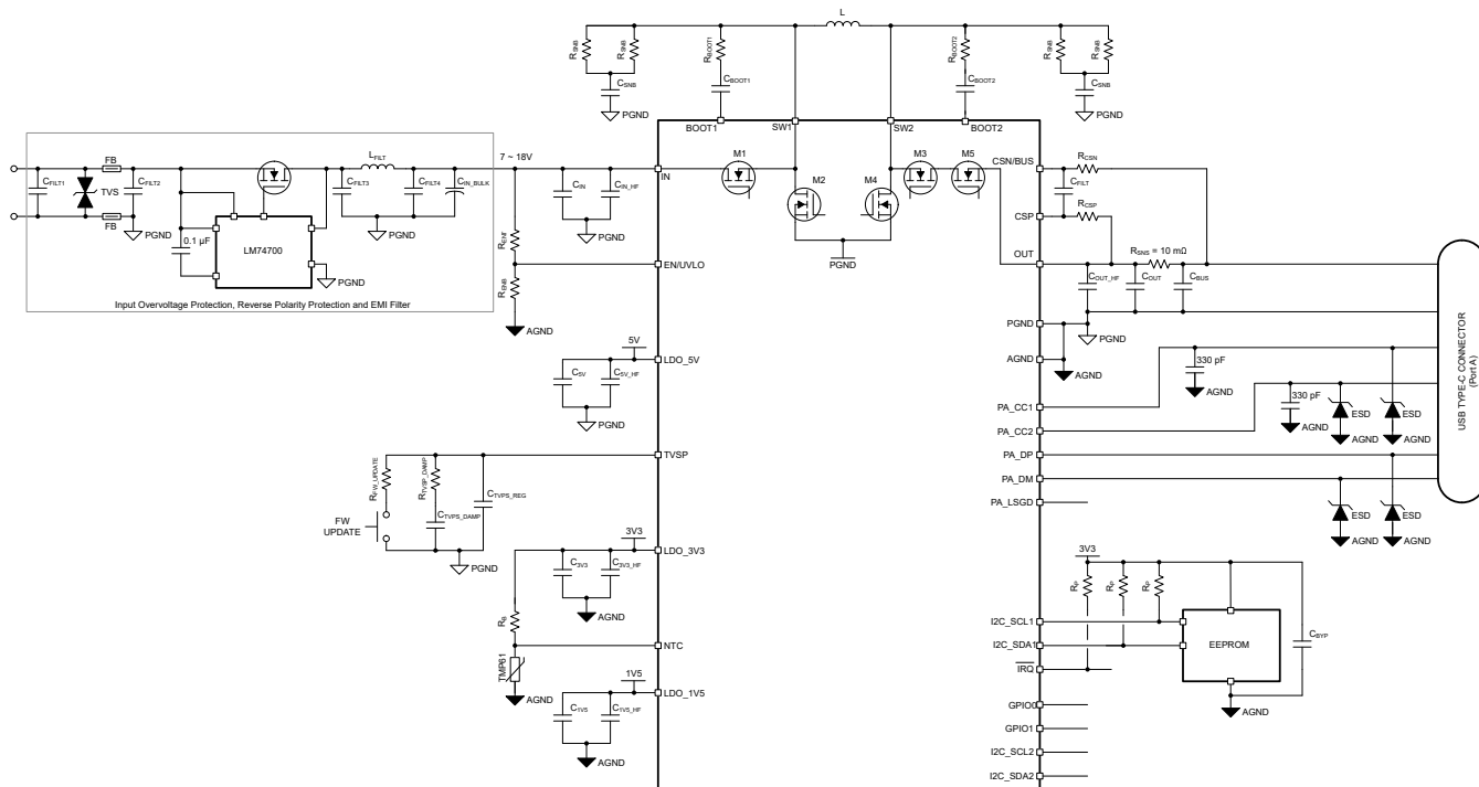
図 9-3. TPS25762-Q1 のアプリケーション回路図
