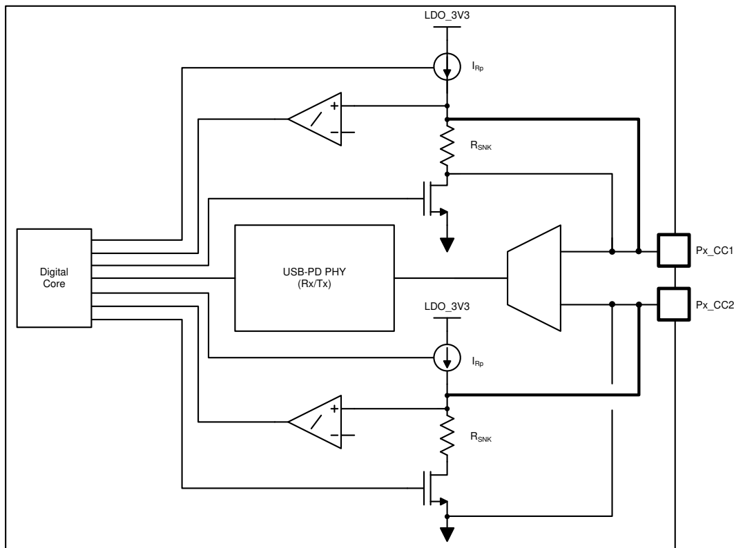
図 8-18. USB-PD 物理層およびプラグと方向の簡素検出回路
