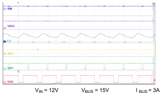
図 9-26. 昇降圧モード : 公称 V_{IN} 、3A 負荷
