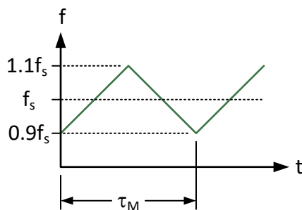
図 8-13. 三角波変調を使用したディザリング
