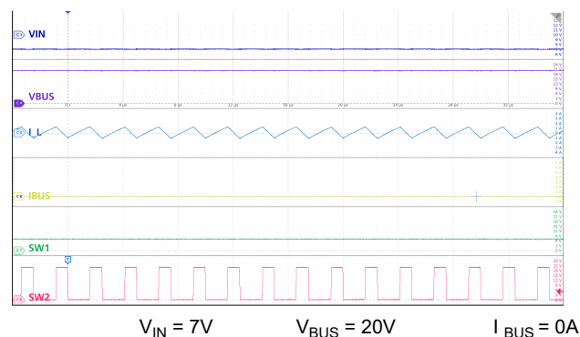
図 9-14. 昇圧モード：低 V_{IN} 、無負荷
