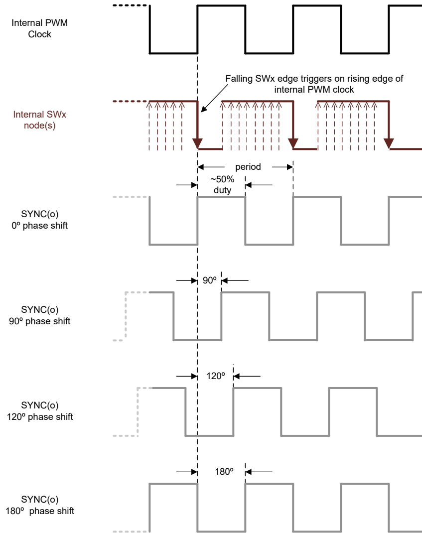
図 8-14. SYNC(o) 位相シフト
