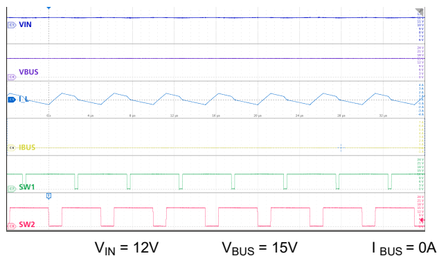
図 9-25. 昇降圧モード : 公称 V_{IN} 、無負荷
