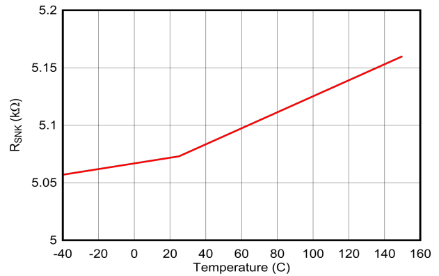
図 6-38. Type-C ケーブル検出 : R_{SnK} と温度との関係
