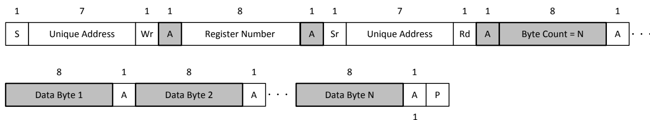
図 8-39. I 2 C 固有アドレス読み取りレジスタ プロトコル
