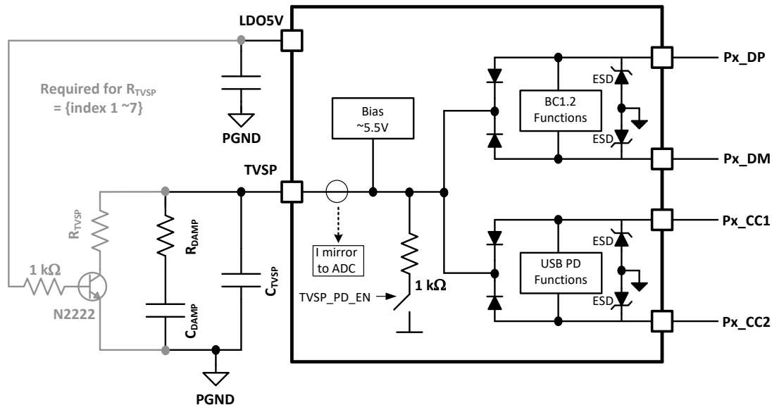
図 8-5. R TVSP の回路構成
