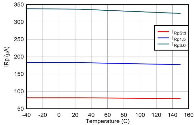
図 6-37. Type-C ケーブル検出 : I_{Rp} と温度との関係
