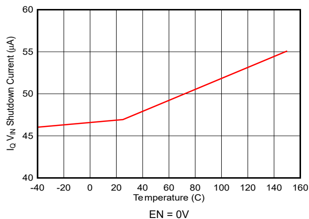
図 6-1. I_Q V_{IN} のシャットダウン電流と温度との関係
