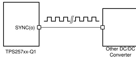
図 8-15. SYNC(o) を使用した外部 DC/DC コンバータの駆動
