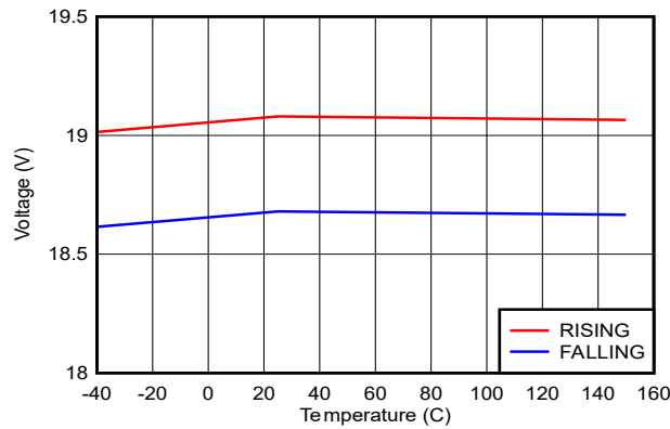
図 6-7. V_{IN(OVP)} と温度との関係
