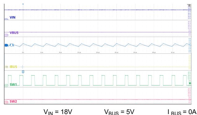
図 9-15. 降圧モード：高 V_{IN} 、無負荷
