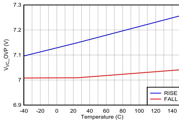
図 6-41. Type-C ケーブル検出、 V_{CONN} : 過電圧保護スレッシュホールドと温度との関係
