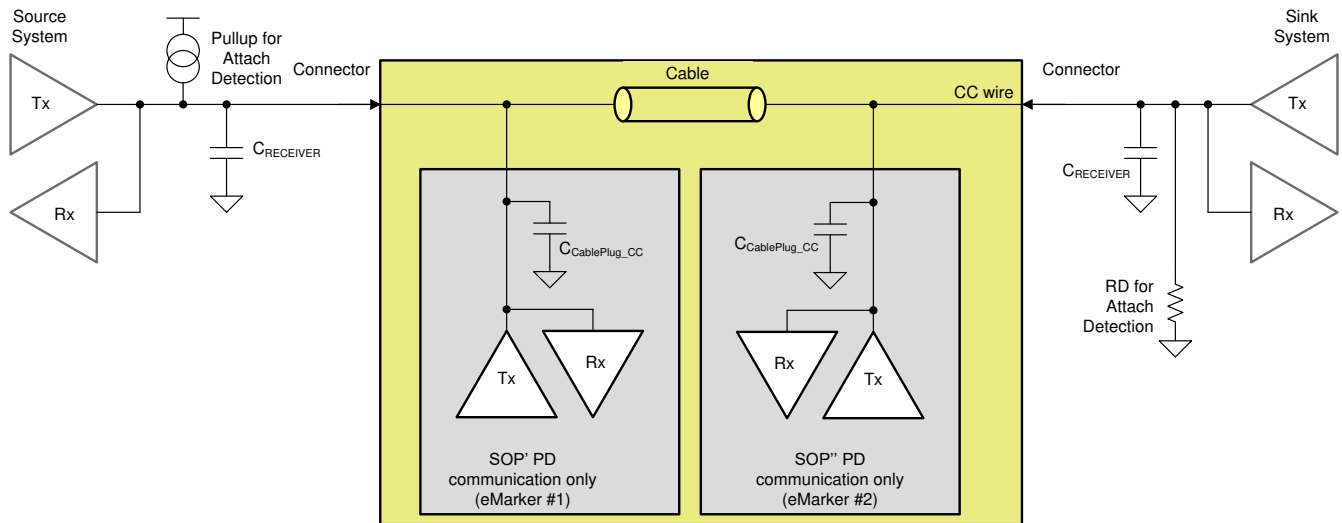
図 8-25. USB-PD マルチドロップ構成の例
