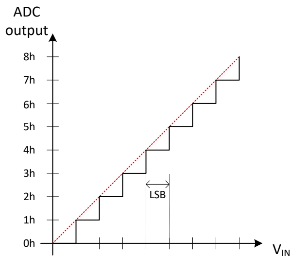
図 8-31. ADC 変換
