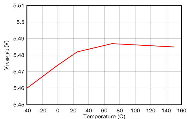
図 6-14. V_{TVSP\_PU} と温度との関係
