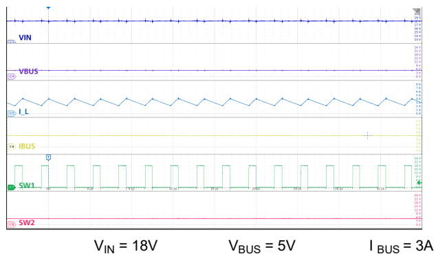
図 9-17. 降圧モード：高 V_{IN} 、3A 負荷
