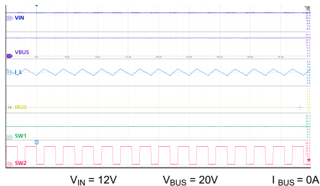
図 9-18. 昇圧モード：公称 V_{IN} 、無負荷
