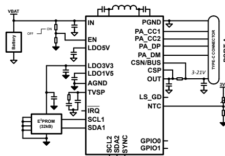
TPS25762-Q1 のアプリケーション概略図
