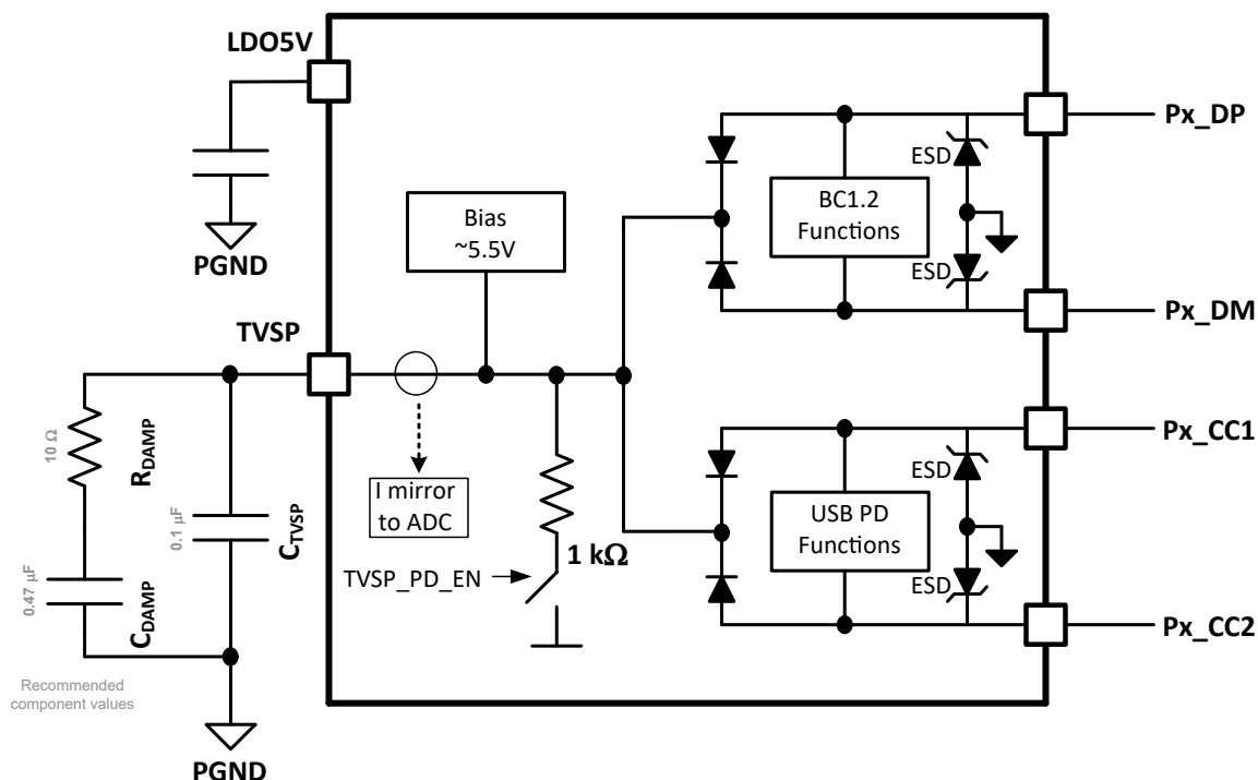
図 8-4. 基本的な TVSP ピン接続
