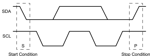
図 8-35. I 2 C の START 条件と STOP 条件の定義
