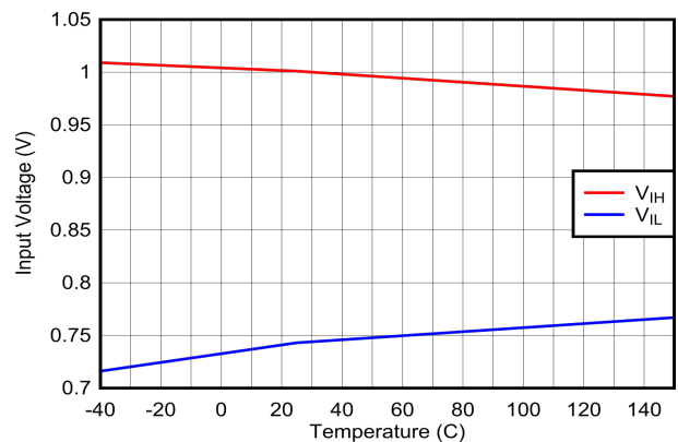
図 6-48. GPIO : 入力電圧スレッシュホールドと温度との関係
