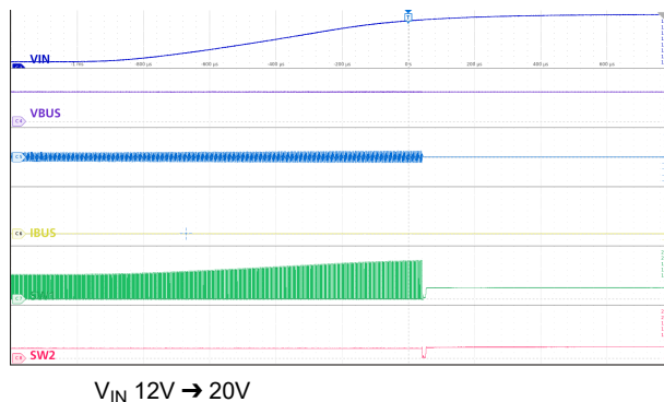
図 9-27. V_{IN(OVP)} 進入
