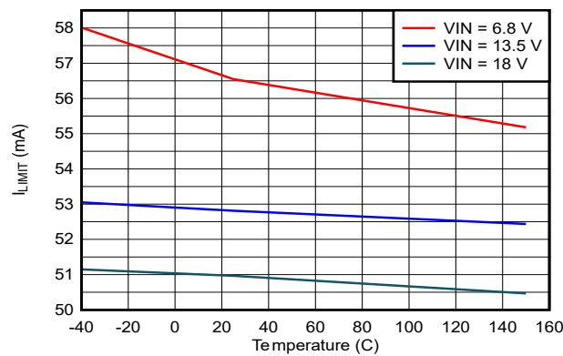
図 6-11. LDO_3V3 電流制限、 V_{IN} と温度との関係
