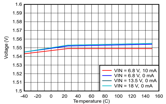
図 6-12. LDO_1V5、 V_{IN} と温度との関係
