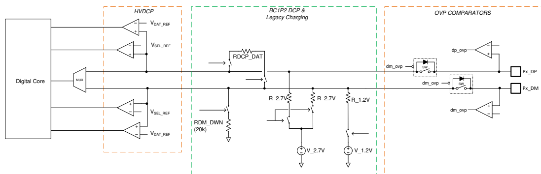
図 8-32. BC1P2 の機能図
