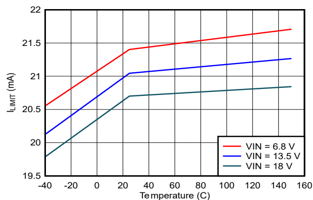
図 6-13. LDO_1V5 電流制限、 V_{IN} と温度との関係
