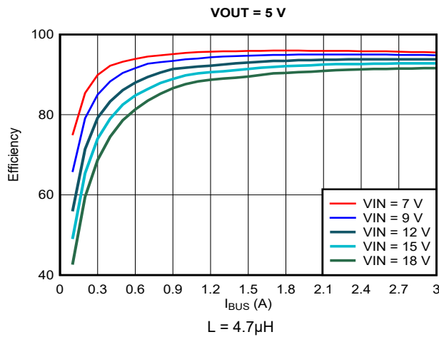
図 9-6. 効率と出力電流 ( I_{OUT} )、 V_{OUT} = 5V との関係
