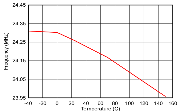
図 6-35. (M0) 24MHz 発振器と温度との関係
