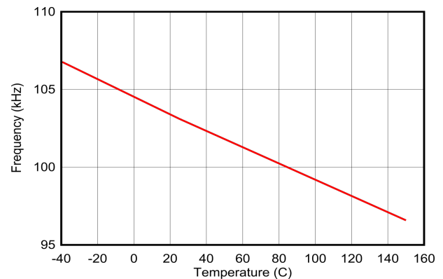
図 6-36. (M0) 100kHz 発振器と温度との関係
