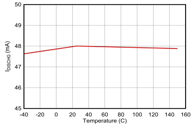
図 6-34. V_{BUS} 放電電流と温度との関係
