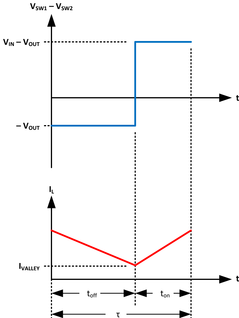
図 8-8. 降圧状態
