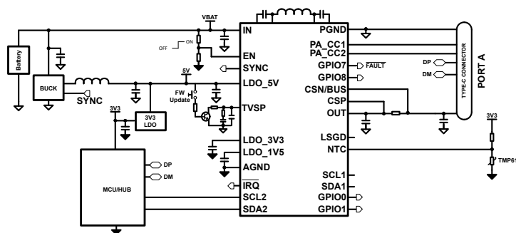
図 9-2. マイコン / ハブ搭載の簡易シングル USB PD
