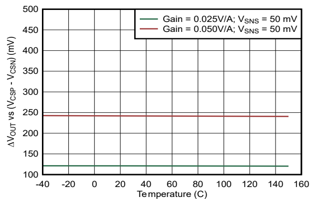
図 6-30. ケーブル電圧ドロップ補償と温度との関係
