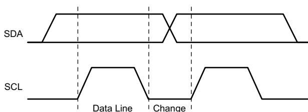
図 8-36. I 2 C ビット転送
