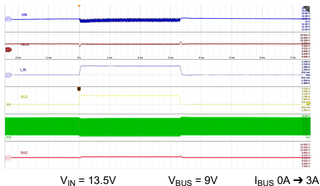
図 9-31. 負荷過渡 (降圧) : V BUS = 9V
