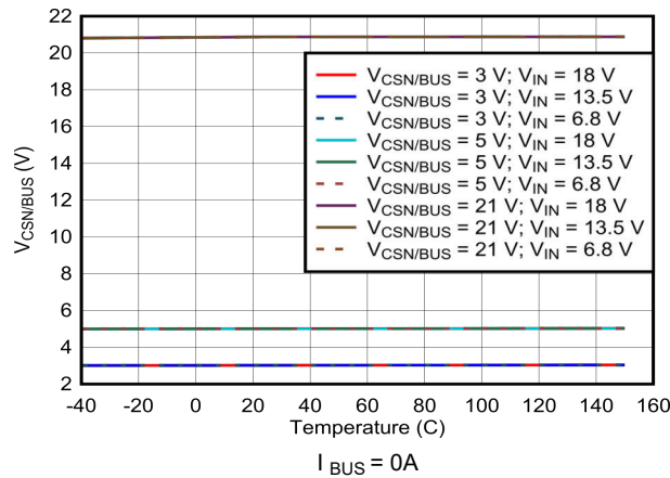
図 6-33. 昇降圧出力電圧レギュレーションと温度との関係
