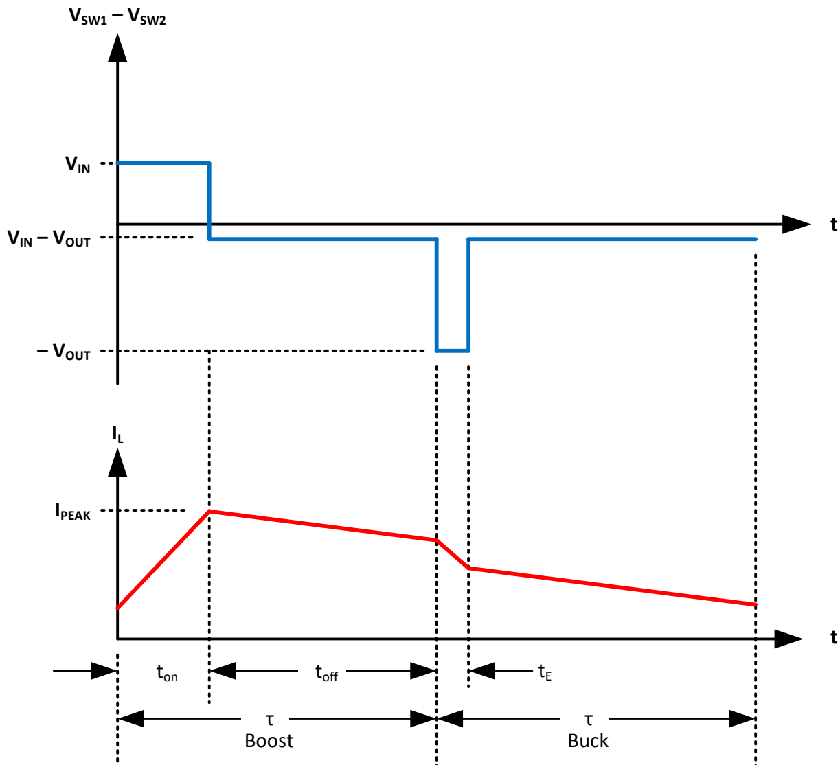
図 8-10. 昇圧遷移
