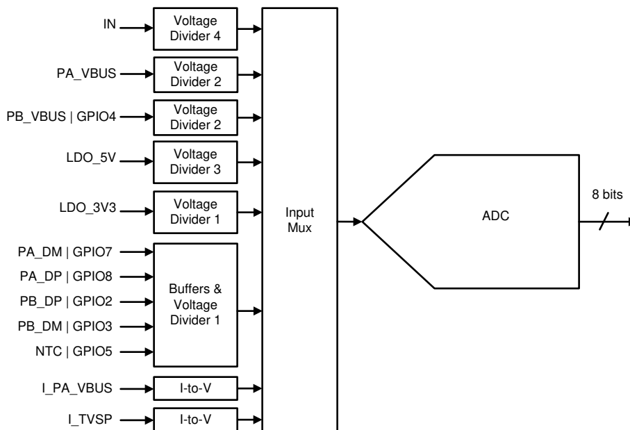
図 8-30. SAR ADC
