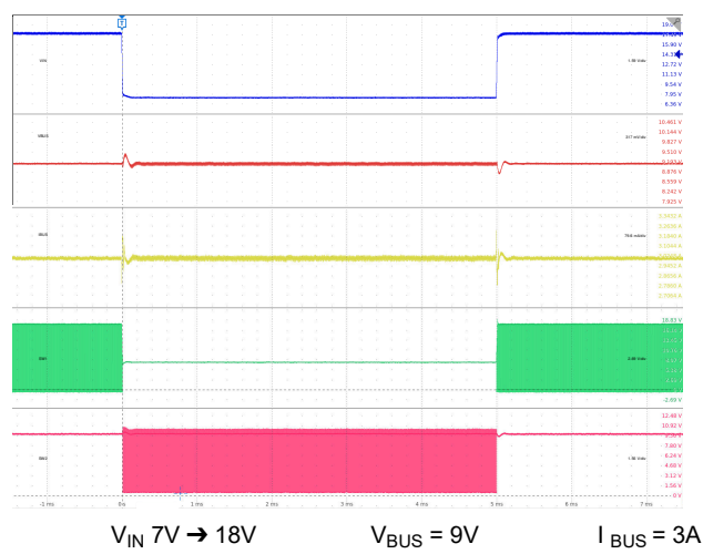
図 9-37. ライン過渡： V_{BUS} = 9V
