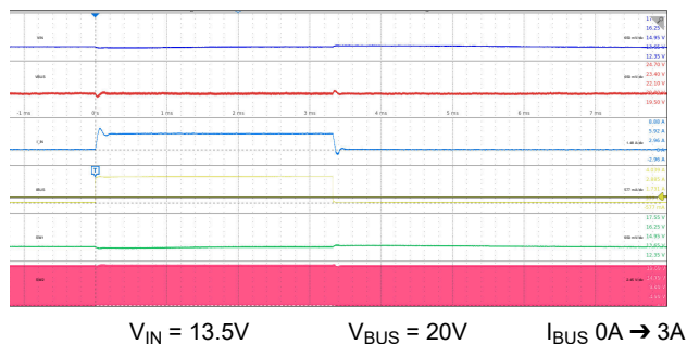
図 9-33. 負荷過渡 (昇降圧) : V BUS = 20V
