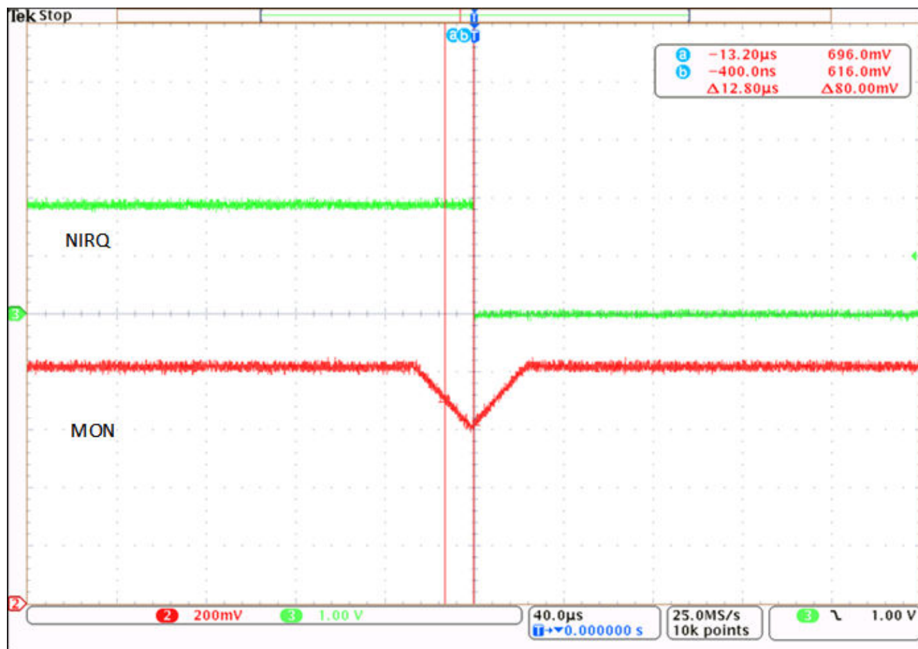
図 9-5. NIRQ は 12.8μs UV デバウンス フィルタによって低電圧フォルトでトリガされます
