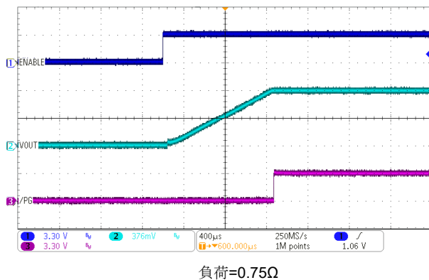
図 9-21. EN ピンを使用したスタートアップ
