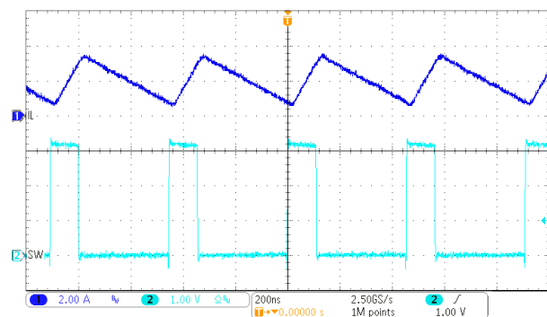
図 9-16. PWM-CCM 動作
