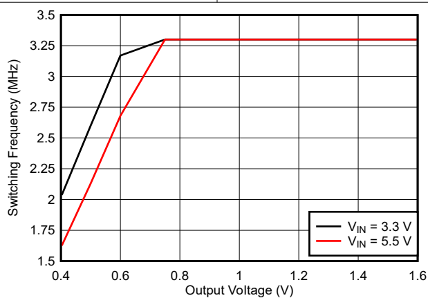
図 6-5. 最大スイッチング周波数と V_{IN} および V_{OUT} との関係
