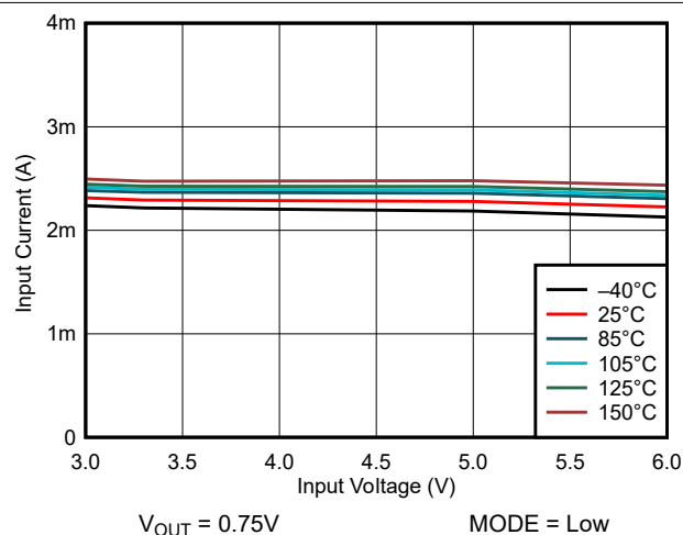
図 6-1. 動作電源電流 (パワーセーブモード)
