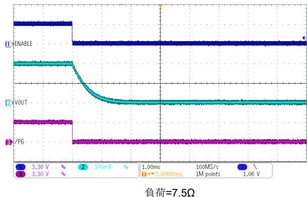
図 9-22. EN ピンを使用したシャットダウン (放電イネーブル)
