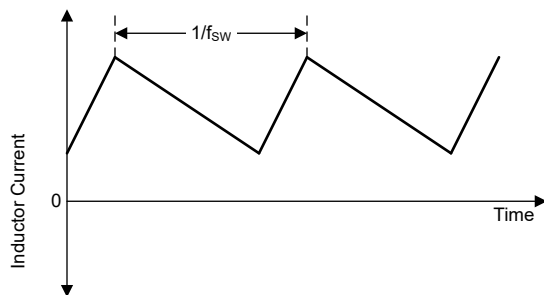
図 7-2. 連続導通モード (PWM-CCM) 電流波形
