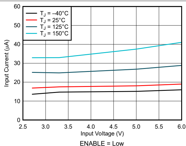
図 6-3. 静止電源電流
