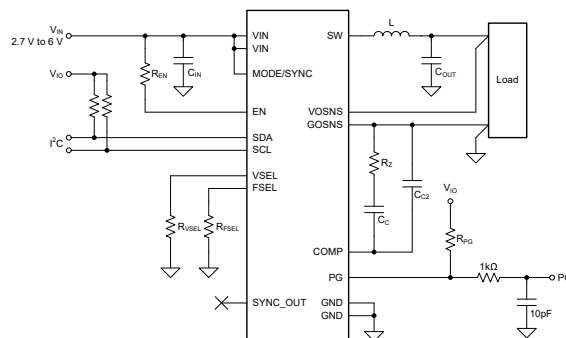
TPS6287x-Q1 の概略回路図
