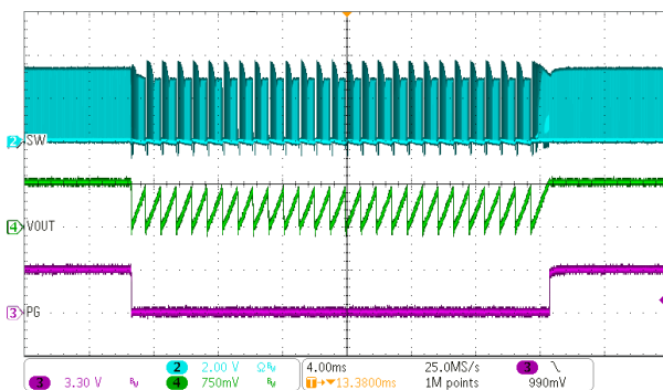
図 9-24. 電流制限 (ヒカップ)
