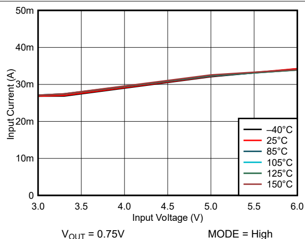
図 6-2. 動作電源電流 (強制 PWM)
