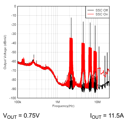
図 9-19. スペクトラム拡散動作
