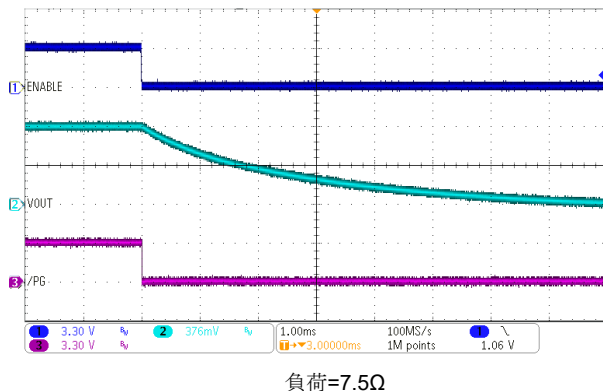
図 9-23. シャットダウン (放電ディスエーブル)
