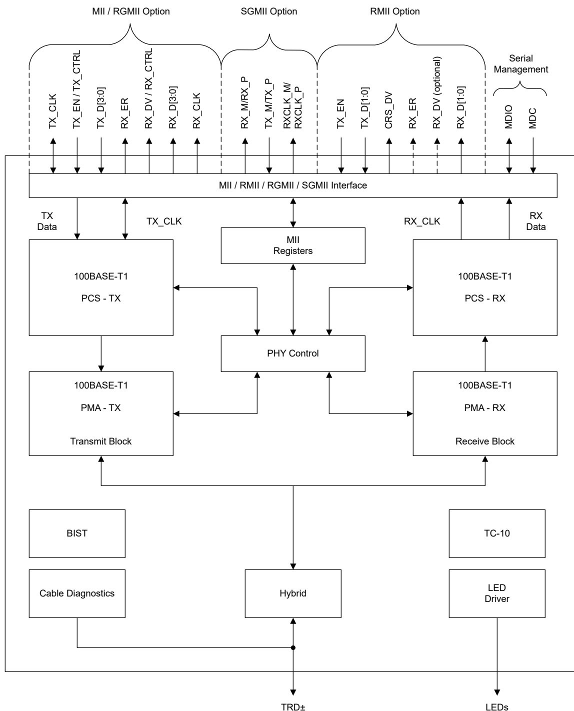
図 7-1. DP83TC813S-Q1
