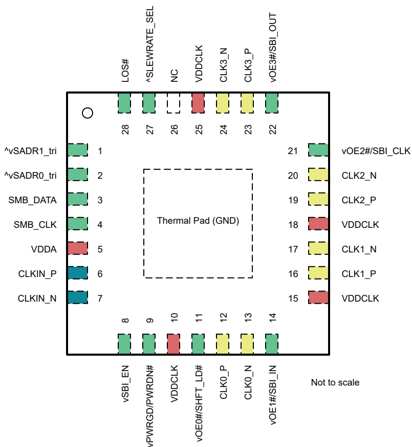
図 5-4. LMKDB1104 および LMKDB1104FS 4mm × 4mm VQFN パッケージ 28 ピン 上面図
