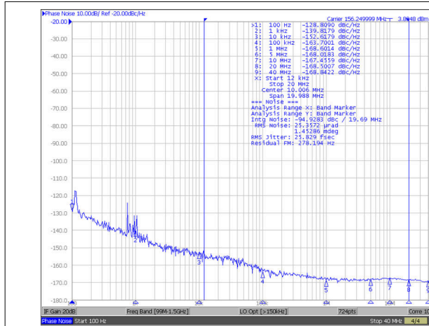
図 6-3. 156.25MHz における入力ソース (12kHz - 20MHz)
