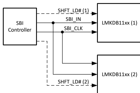
図 8-13. SBI スタート ポロジ
