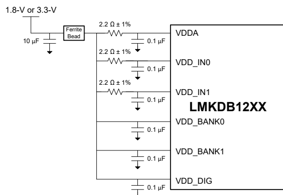
図 10-5. LMKDB12XX マルチプレクサの電源に関する推奨事項
