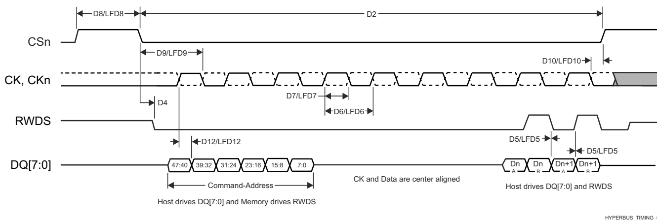
図 6-69. HyperBus タイミング図 – 受信モード
