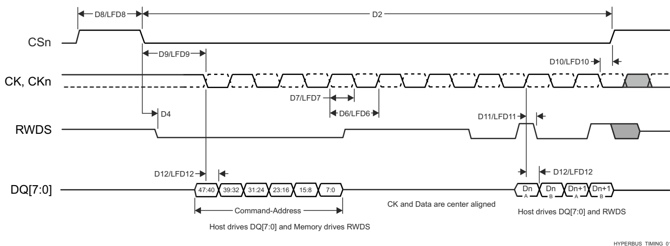
図 6-68. HyperBus タイミング図 – 送信モード
