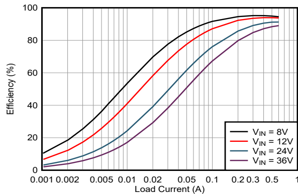
図 8-2. 効率
