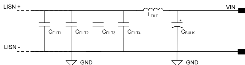
図 8-29. 標準入力 EMI フィルタ回路図
