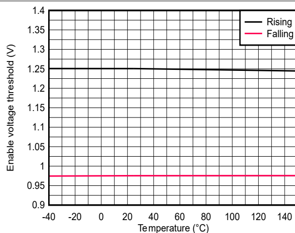
図 6-8. イネーブル スレッシュリッド電圧
