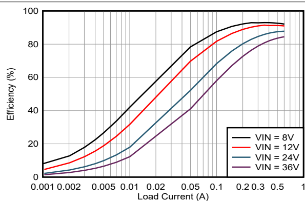
図 8-6. 効率
