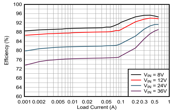
図 8-3. 効率
