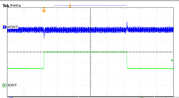
図 8-15. シャットダウン
