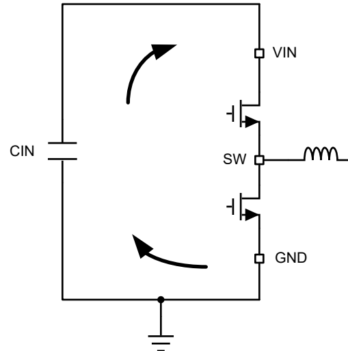
図 8-31. 高速過渡を持つ電流ループ
