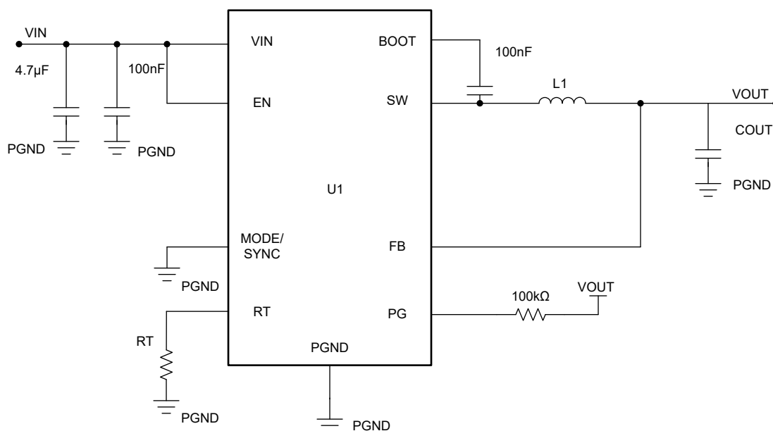
図 8-30. アプリケーション回路例
