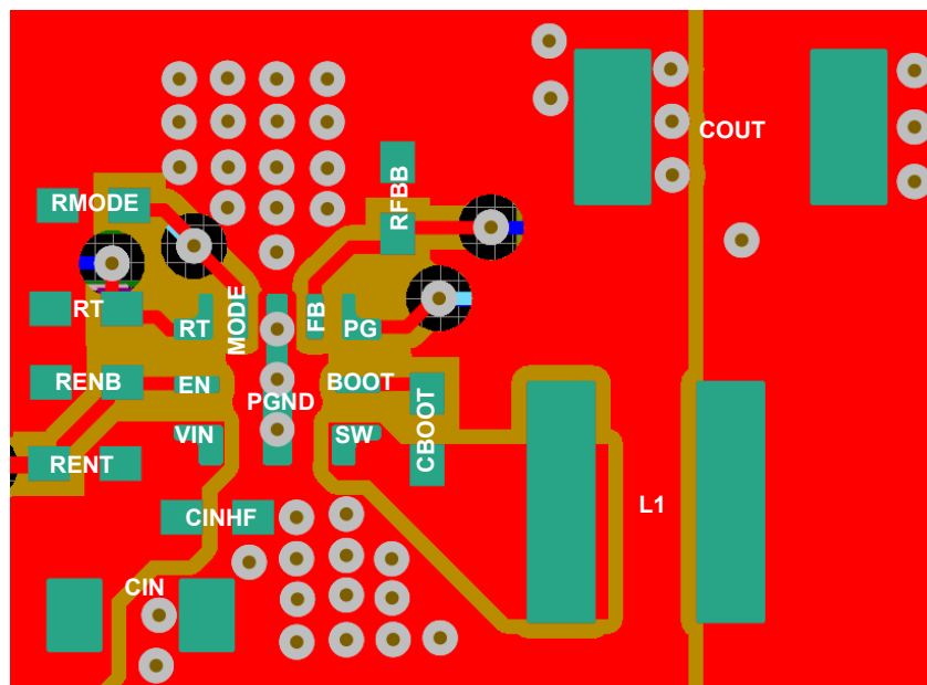
図 8-32. レイアウト例
