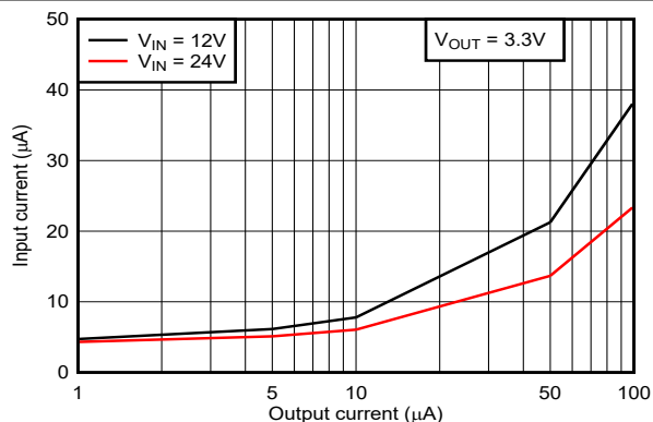
図 8-13. 軽負荷時における入力電流と負荷電流との関係
