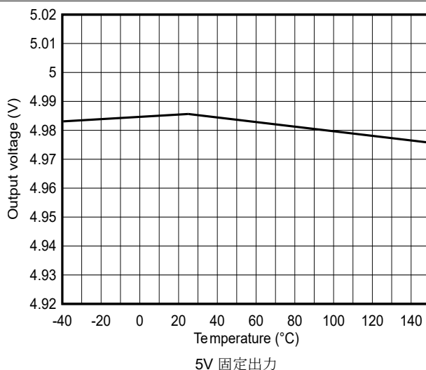
図 6-6. 出力電圧精度
