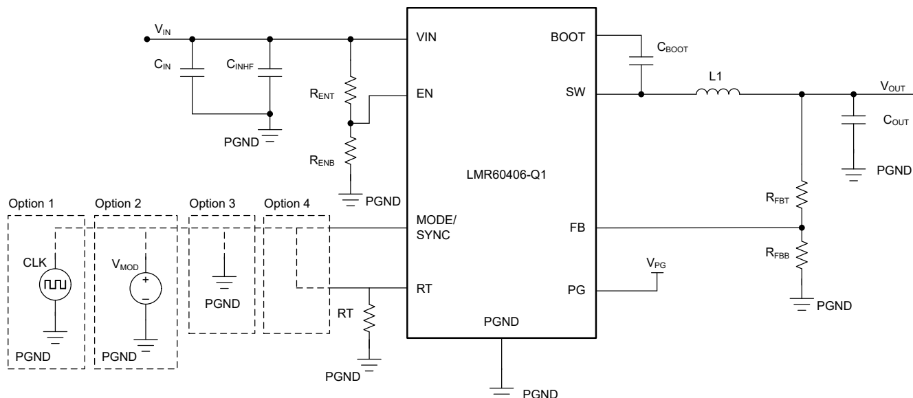
図 8-1. LMR60406-Q1 のリファレンス回路図
