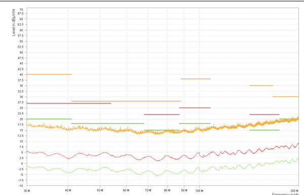
V_{OUT} = 3.3V F_{SW} = 2MHz I_{OUT} = 1A 周波数スパン: 30MHz ~ 200MHz
