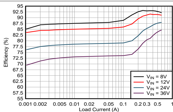
図 8-7. 効率
