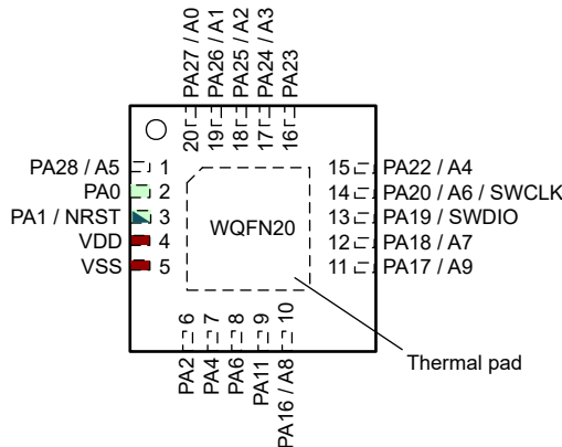
図 6-3. 20 ピン RUK (WQFN) (上面図)
