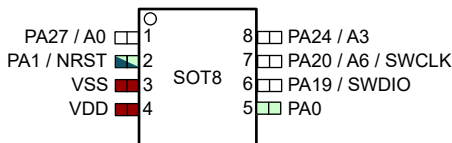
図 6-5. 8 ピン DDF (SOT) (上面図)
