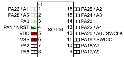
図 6-4. 16 ピン DYY (SOT) (上面図)
