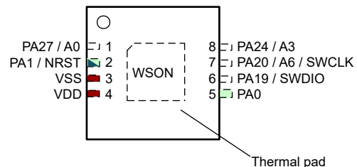
図 6-6. 8 ピン DSG (WSON) (上面図)
