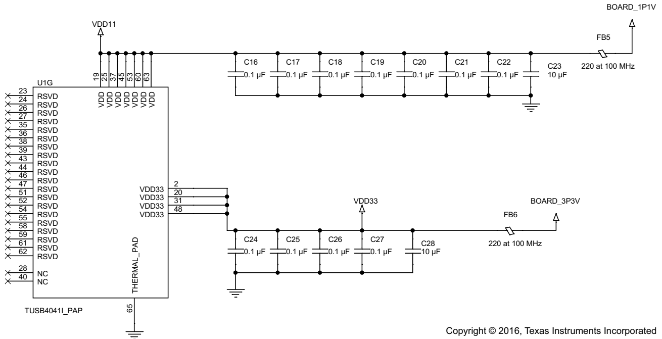
図 7-9. TUSB4041I-Q1 電力の実装
