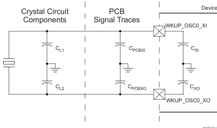
図 6-27. 負荷容量
