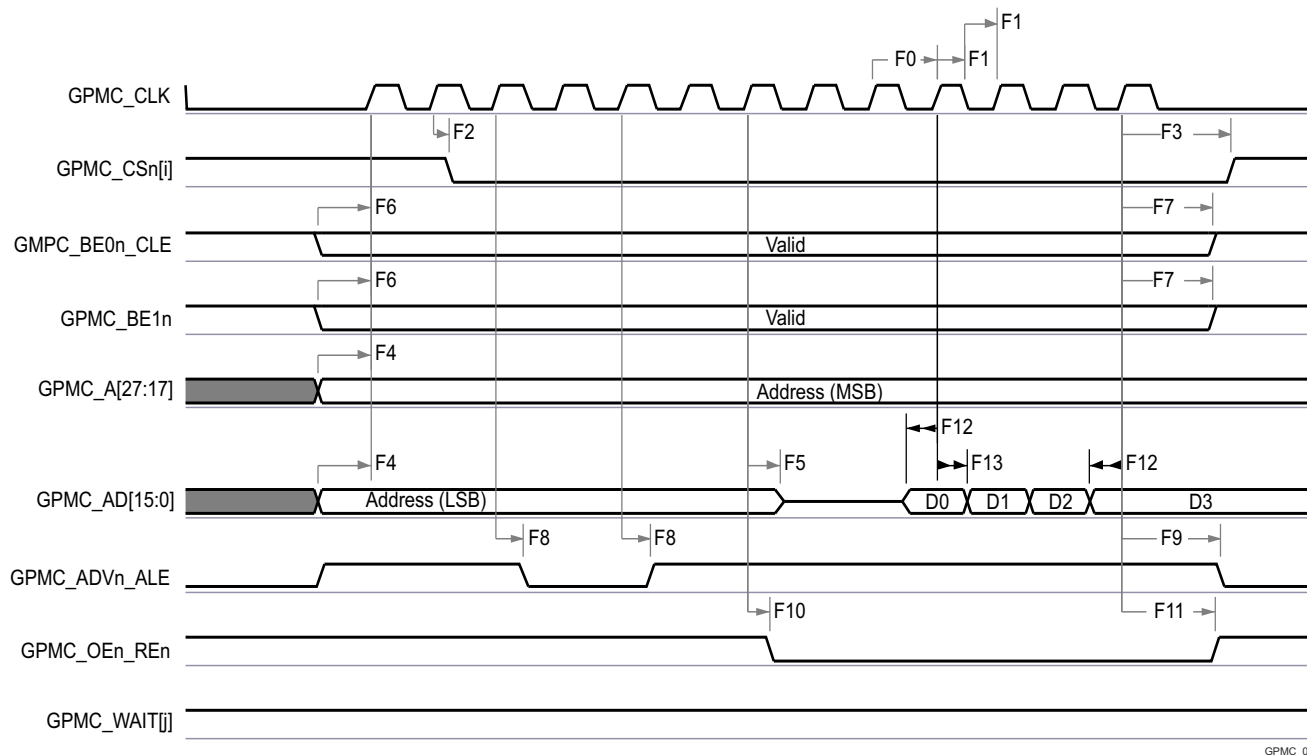
図 6-55. GPMC および NOR フラッシュ — 同期バースト書き込み (GPMCCLKDIVIDER = 0)
