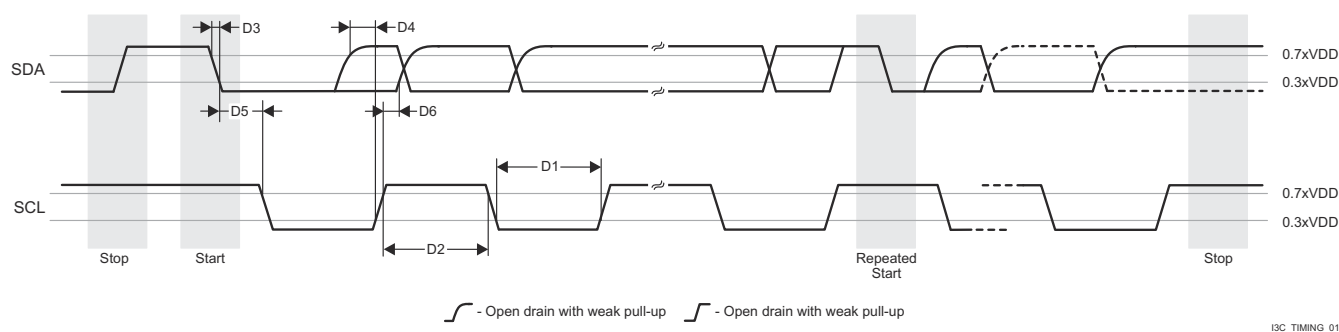
図 6-71. I3C オープン ドレインのタイミング
