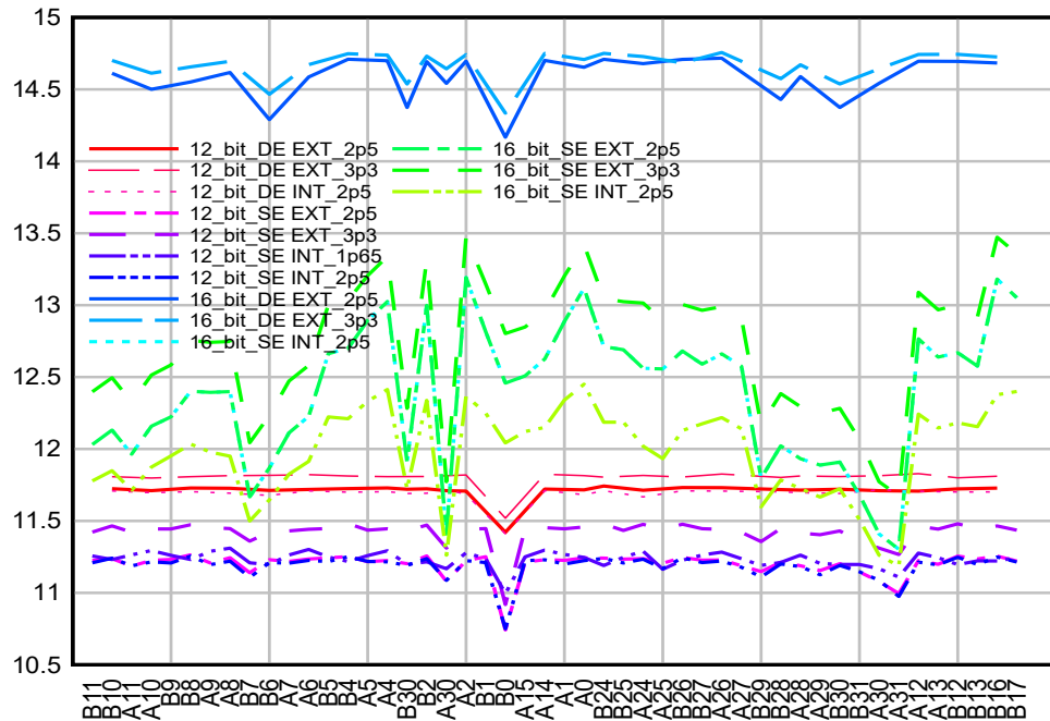
図 6-45. 256 ピン ZEX のチャンネルあたりの ENOB – ADC チャンネル A および B
