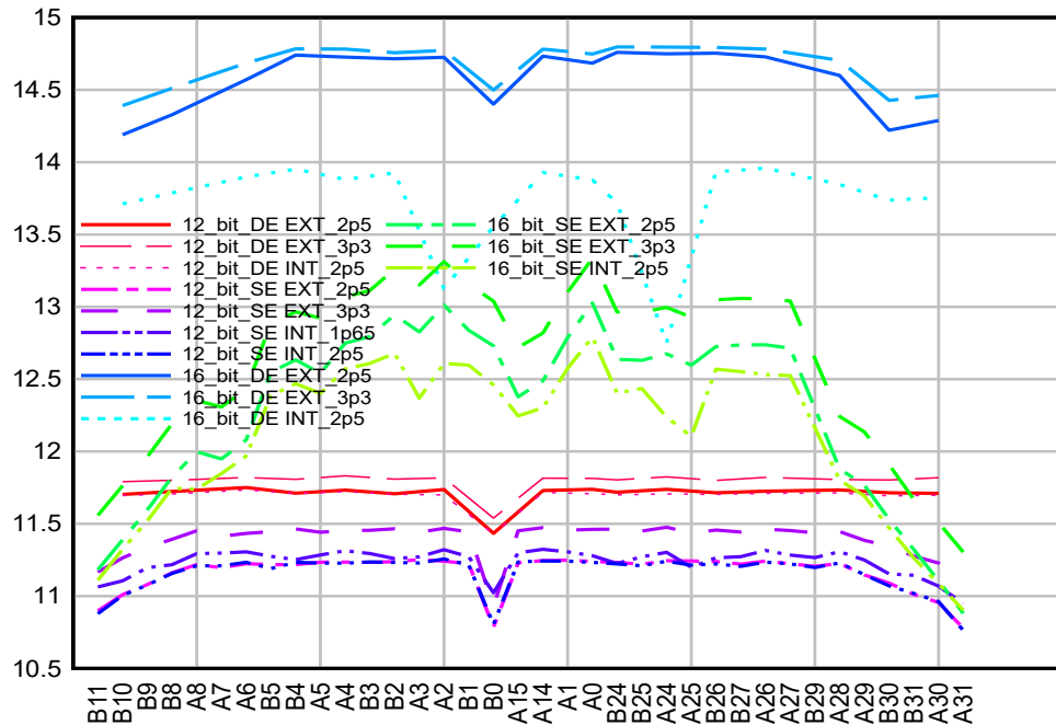
図 6-41. 144 ピン RFS のチャンネルあたりの ENOB – ADC チャンネル A および B
