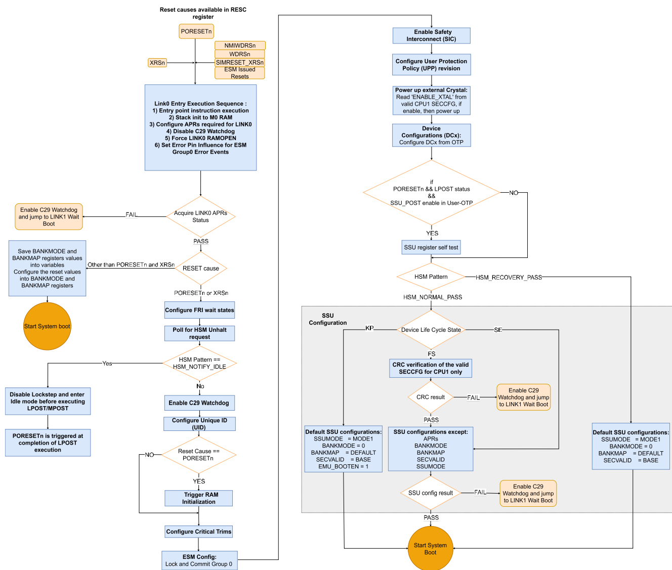
図 7-8. リセットからシステム ブートまでのデバイス ブート フロー
