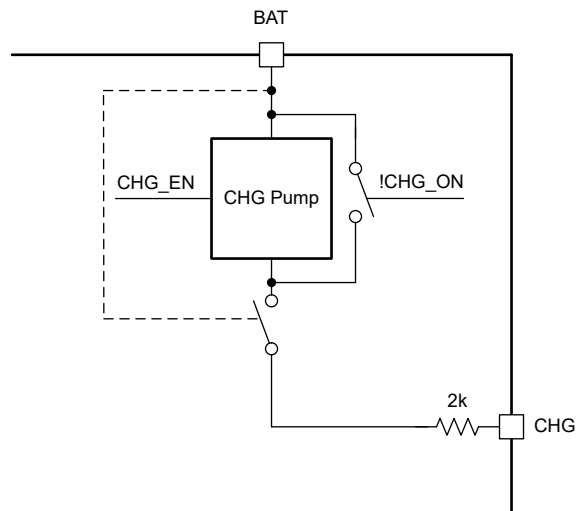
図 5-5. CHG ピン
