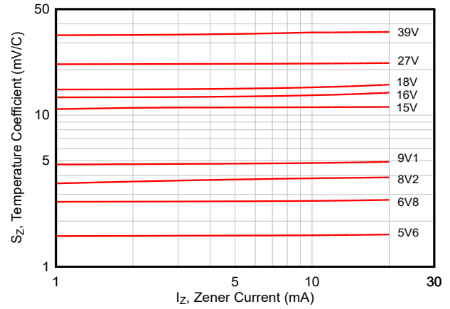
図 5-2. 温度係数
