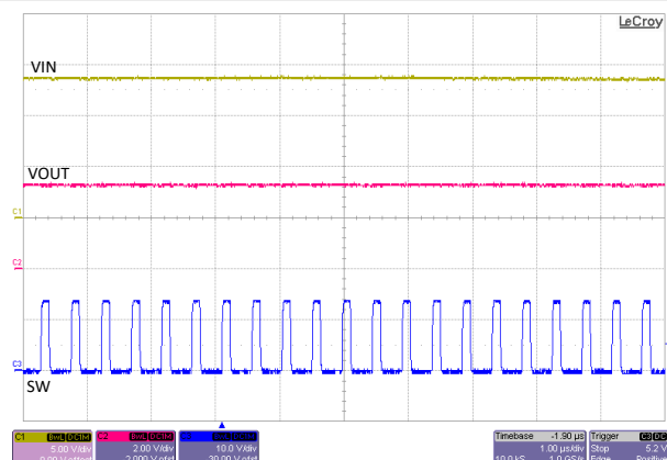
図 8-11. SW ノード、12VIN、3.3VOUT、2.2MHz、2A 負荷電流
