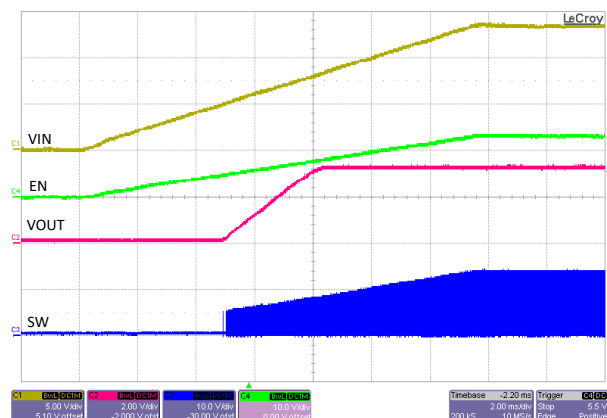
図 8-9. 起動、12VIN、3.3VOUT、2.2MHz、2A 負荷電流
