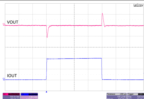
図 8-13. 負荷過渡、12VIN、3.3VOUT、2.2MHz (FPWM)、0A ~ 2A、 1A/\mu s 、 C_{OUT} = 2 \times 22\mu F
