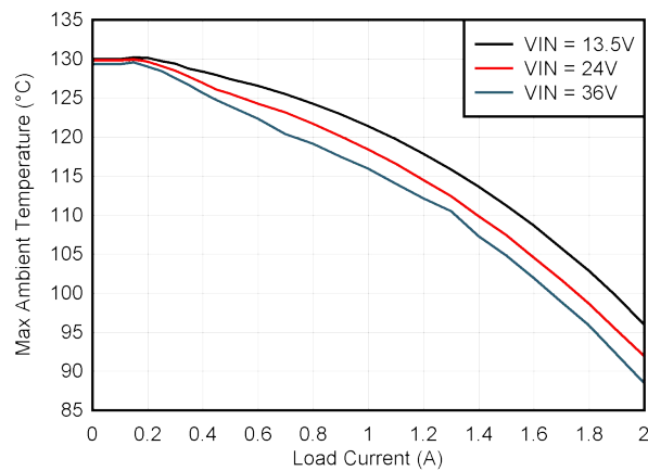
図 8-5. 最大周囲温度と負荷電流との関係 (TPSM33620QEVm の解析)、3.3VOUT、2.2MHz
