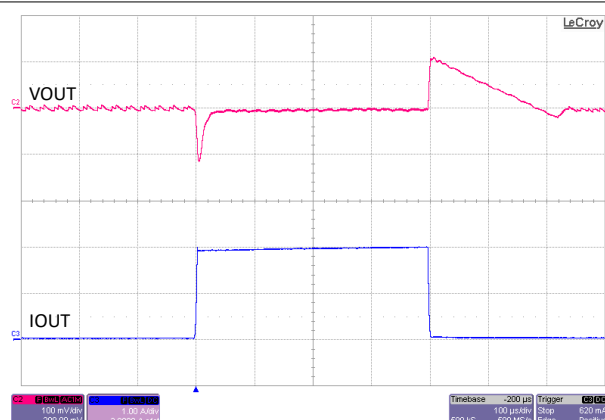
図 8-14. 負荷過渡、12VIN、3.3VOUT、2.2MHz (Auto)、0A ~ 2A へ、 1A/\mu s 、 C_{OUT} = 2 \times 22\mu F
