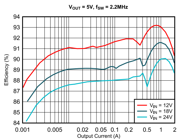
効率と出力電流との関係
