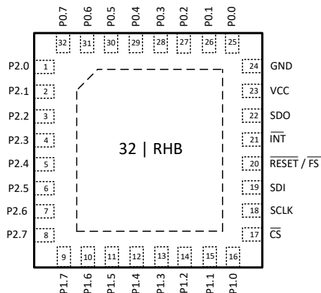
図 4-2. TXE8124-Q1 RHB (VQFN) パッケージ、32 ピン (上面図)
