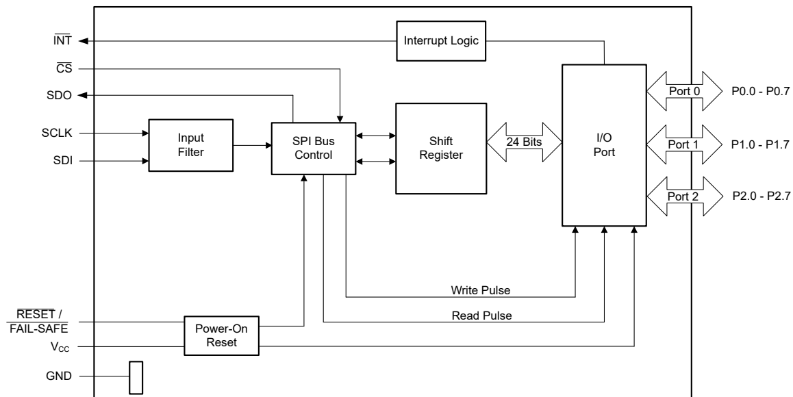
図 7-1. ロジック図
