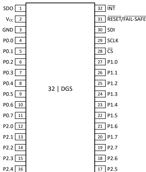
図 4-1. TXE8124-Q1 DGS (VSSOP) パッケージ、32 ピン (上面図)
