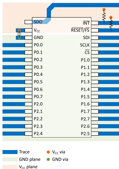
図 8-6. TXE8124-Q1 レイアウト
