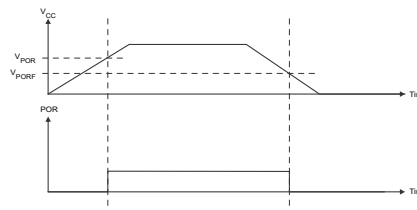
図 8-5. V_{POR}
