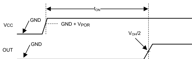
図 6-4. パワーオン リセットのタイミング図
