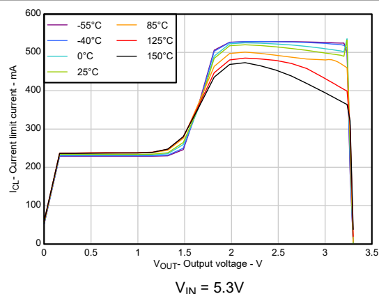
図 5-10. 電流制限と出力電圧との関係
