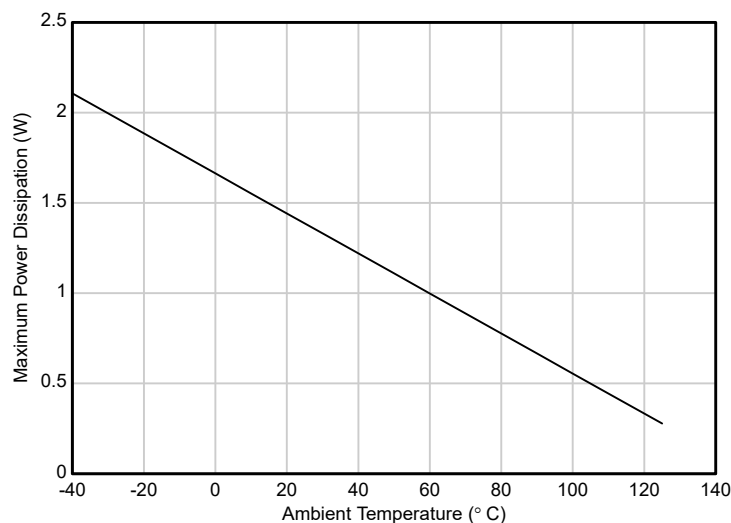
図 7-3. TPS7E82 (DRV) 許容消費電力
