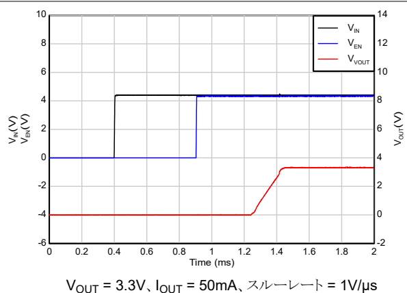
図 7-8. シーケンシングありの起動 (IN の後に EN)
