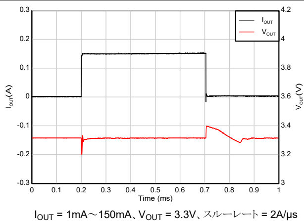
図 7-7. 負荷過渡応答
