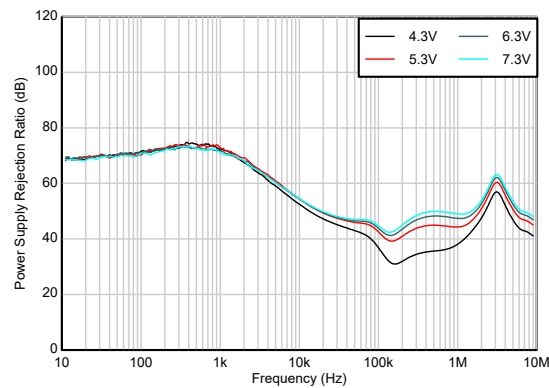
図 5-20. リップル除去と周波数、入力電圧との関係
