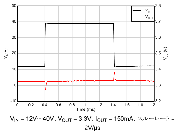
図 7-6. ライト トランジェント
