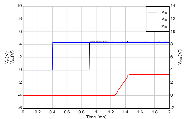
図 5-45. シーケンシングありの起動 (IN の後に EN)
