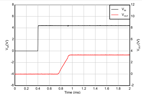
図 5-46. シーケンシングありの起動 (EN の後に IN)
