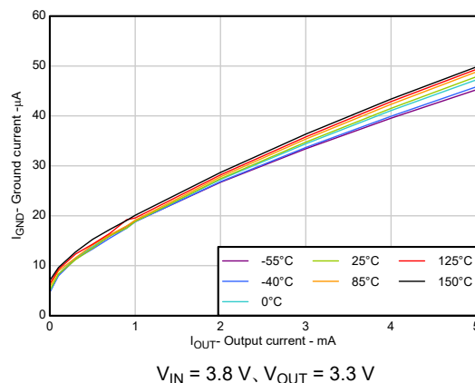
図 5-12. グランド電流と出力電流との関係
