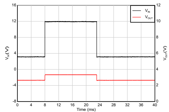
図 5-32. ライン トランジェント
