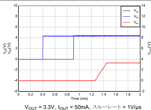
図 7-9. シーケンシングありの起動 (EN の後に IN)
