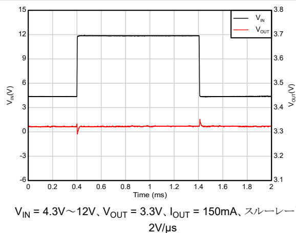
図 5-30. ライン トランジェント
