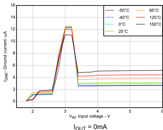
図 5-11. グランド電流と入力電圧との関係
