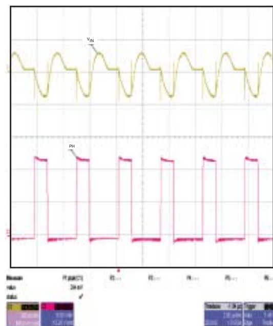
図 20. TPS54233の入力リップル
