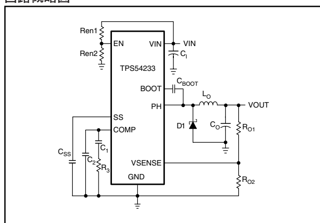
回路概略図
