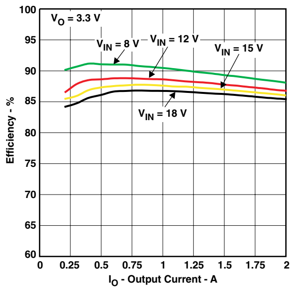
図 14. TPS54233の効率
