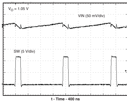
図 13. 入力電圧リップル ( I_O = 2\text{A} )
