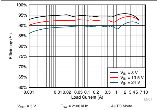
10-11. LM61460-Q1 Efficiency
