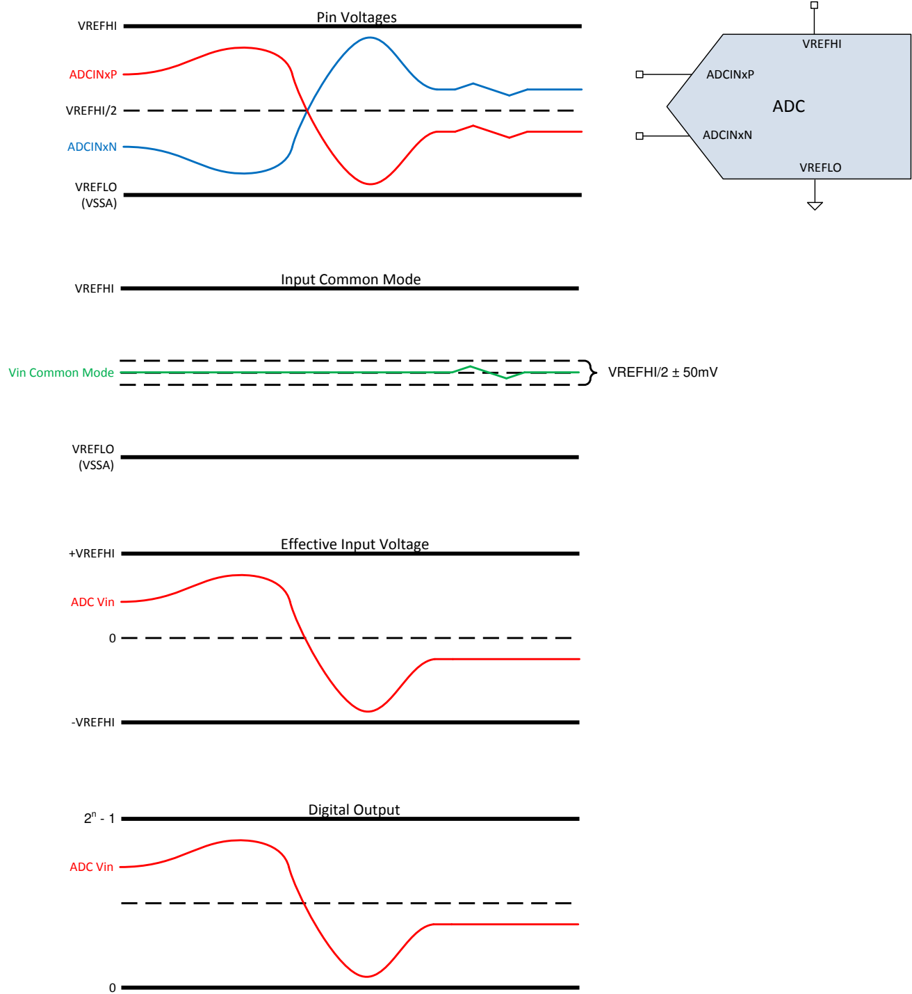
図 6-36. 差動信号モード
