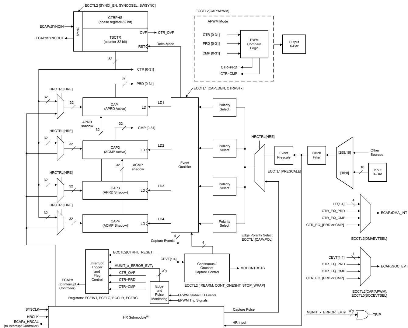
図 6-62. eCAP のブロック図
