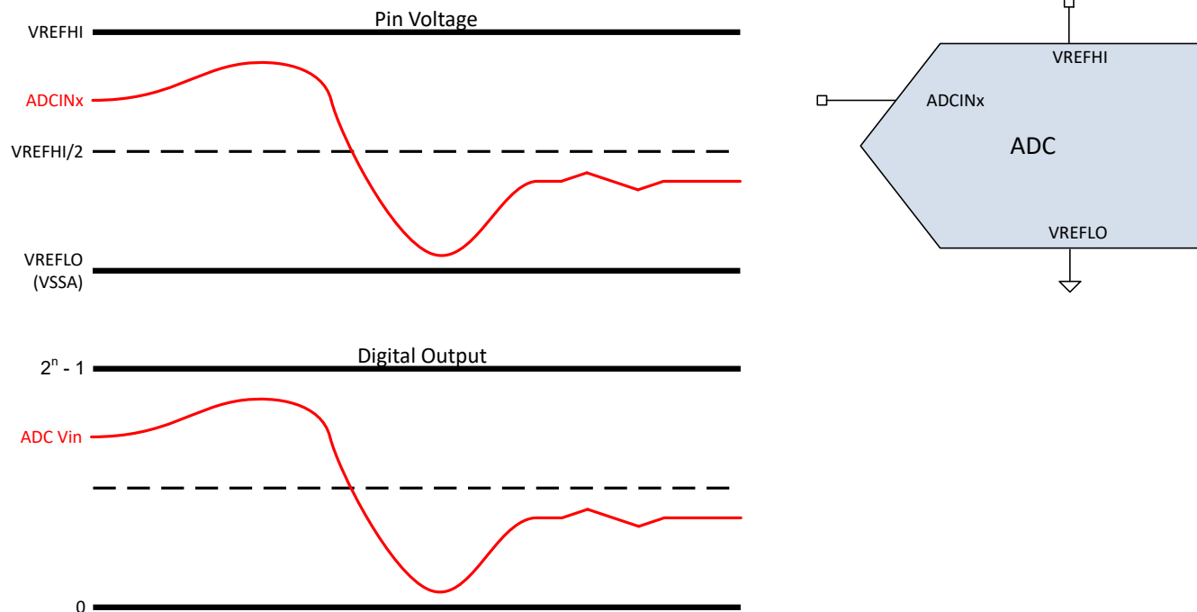
図 6-37. シングルエンド信号モード
