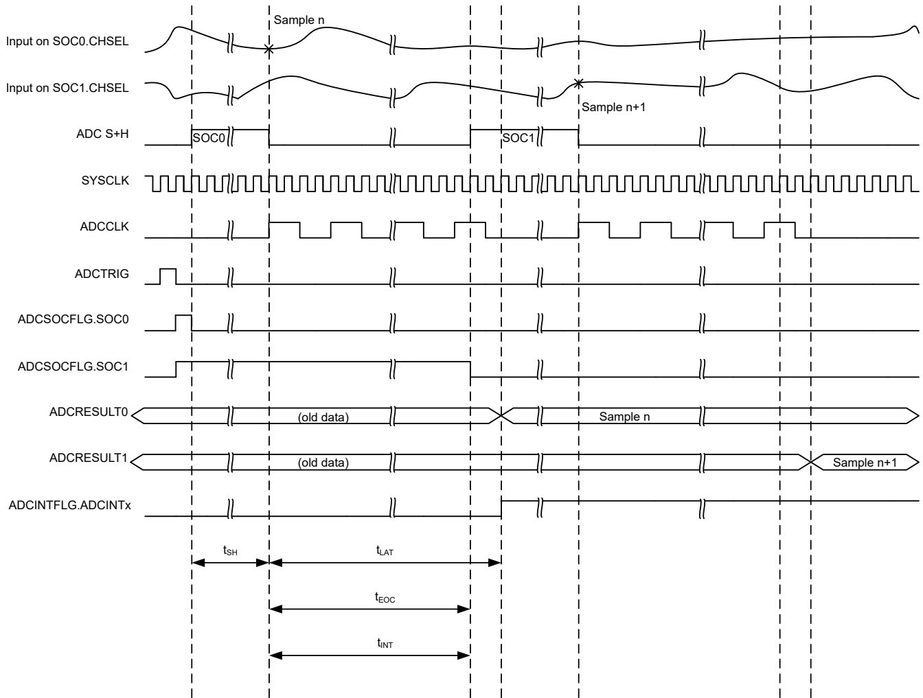
図 6-50. 12 ビット モードの Late 割り込みモードでの ADC タイミング
