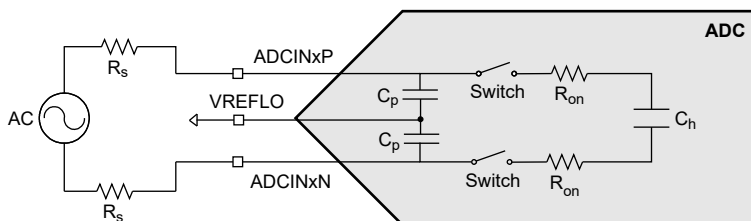
図 6-48. 差動入力モデル
