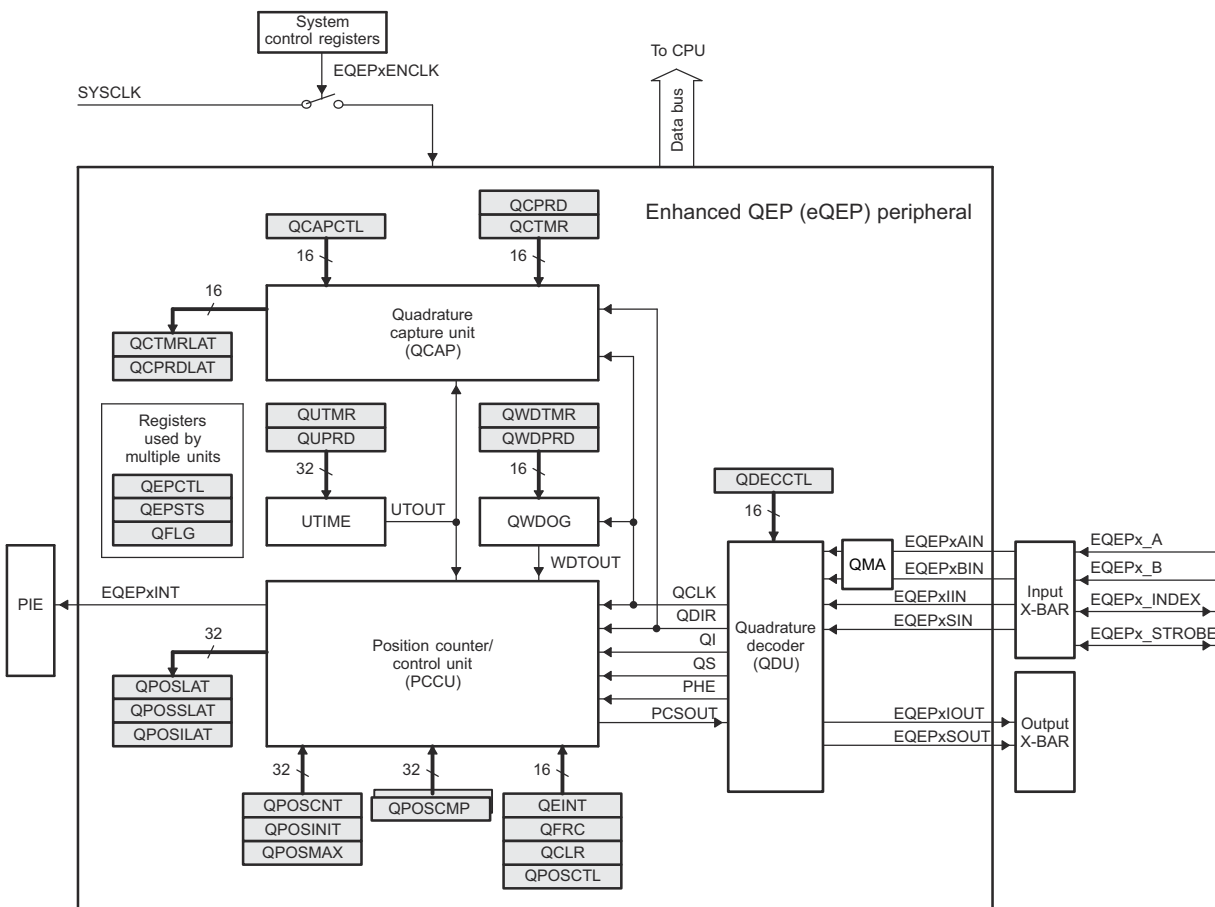
図 6-71. eQEP のブロック図
