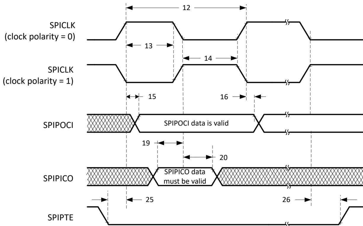
図 6-88. SPI ペリフェラル・モードの外部タイミング (クロック位相 = 0)
