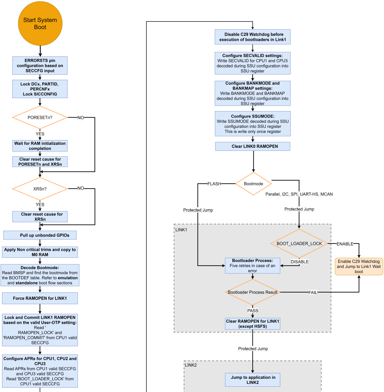
図 7-9. アプリケーション コードまでのシステム ブート フロー
