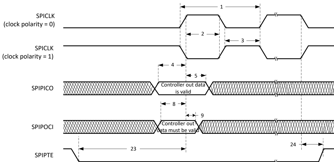
図 6-86. SPI コントローラ・モードの外部タイミング (クロック位相 = 0)
