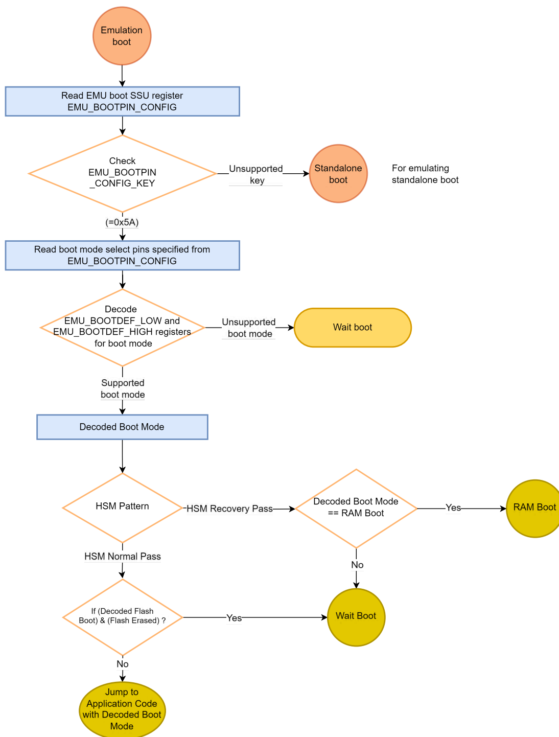
図 7-10. エミュレーションブートフロー
