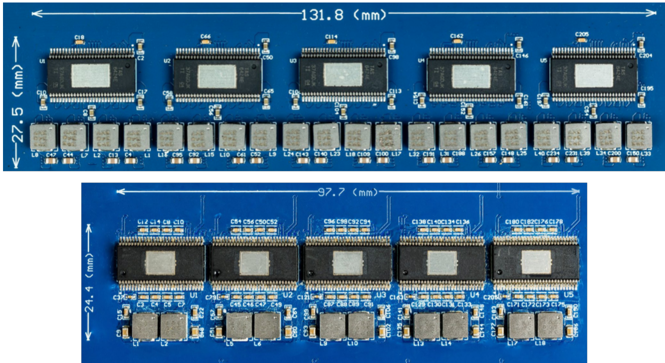
圖 2. 採用 TI 的 TAS6424E-Q1 D 類放大器 (上圖) 的 20 通道汽車音訊系統設計與 TI 的五個 TAS67524-Q1 D 類放大器 (下圖) 相比
