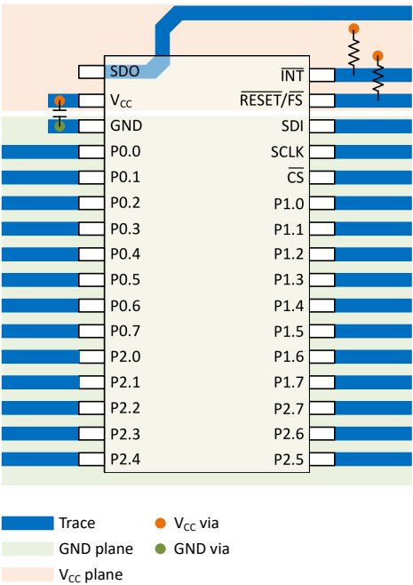
Figure 8-6. TXE8124-Q1 Layout
