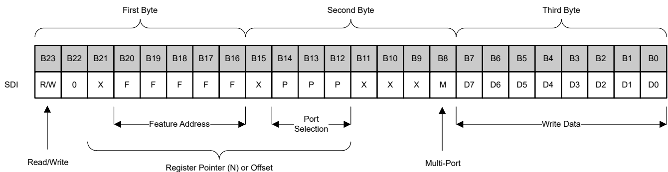
Figure 7-5. TXE8124-Q1 SPI SDI Data Frame Format
