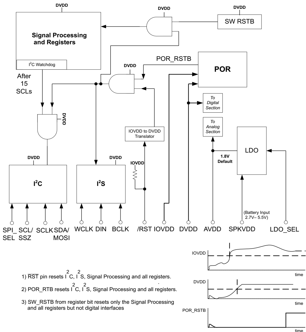
Figure 4-7. POR Diagram
