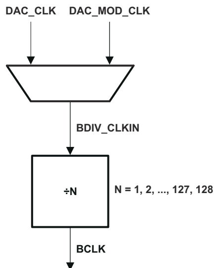
Figure 4-9. BCLK Output Options
