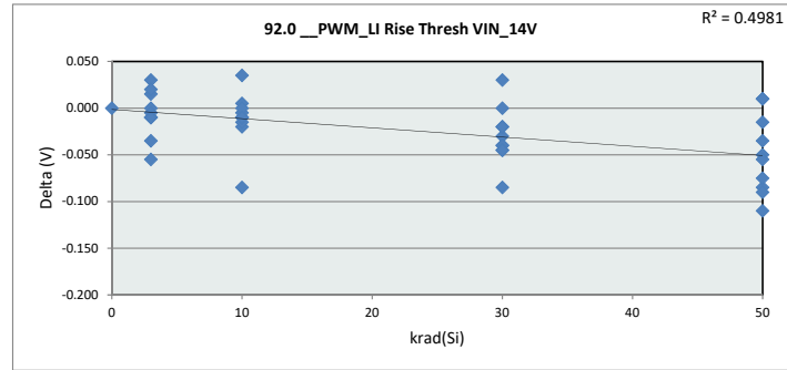
92.0 __PWM_LI Rise
