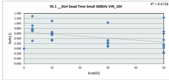
95.1 __DLH Dead Time Small 500kHz VIN_10V
