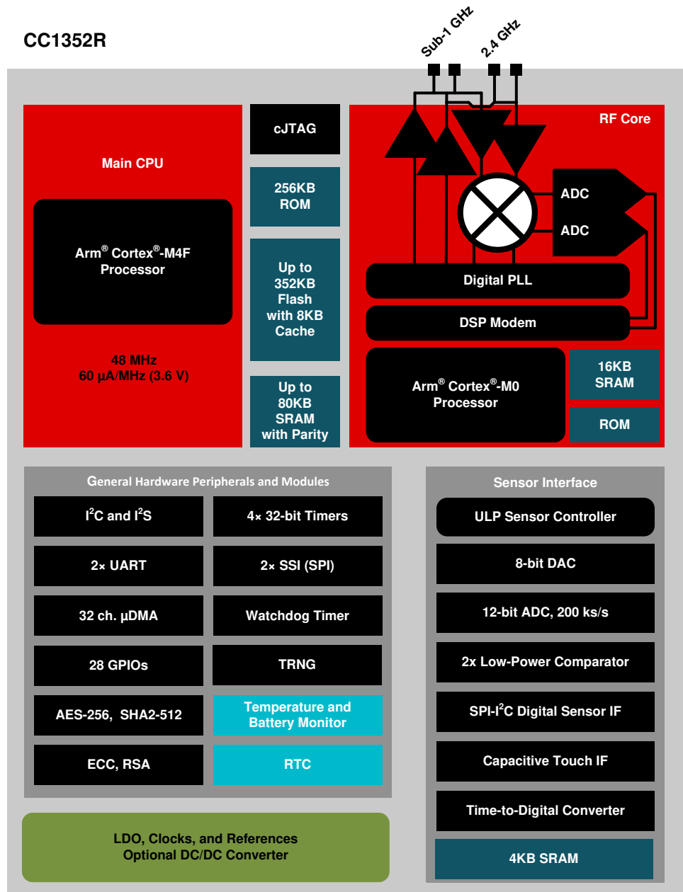
図 4-1. CC1352R Block Diagram
