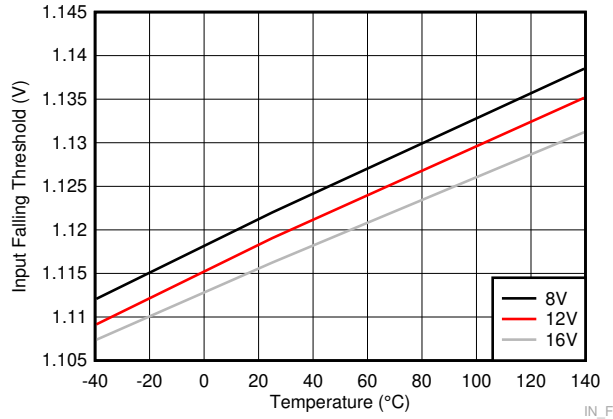
6-8. Input Falling Threshold
