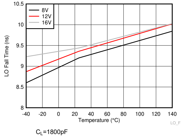
6-17. LO Fall Time
