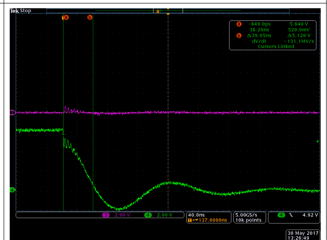
図 8-4. HO Fall Time
