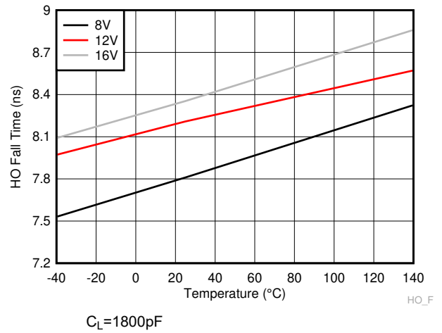
6-19. HO Fall Time
