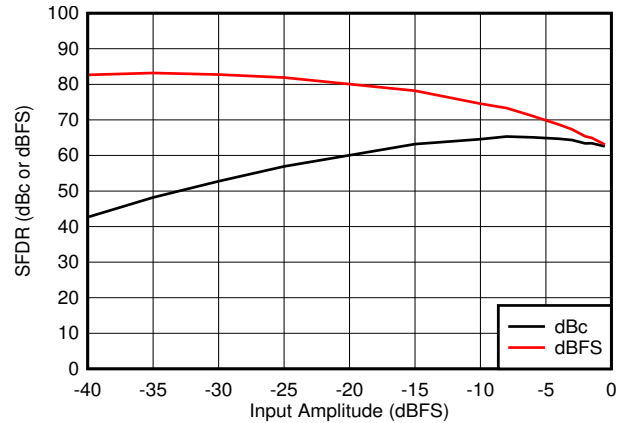
図 5-34. SFDR vs A_{IN}
