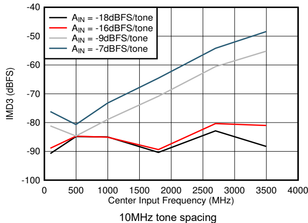
図 5-75. IMD3 vs F_{IN}
