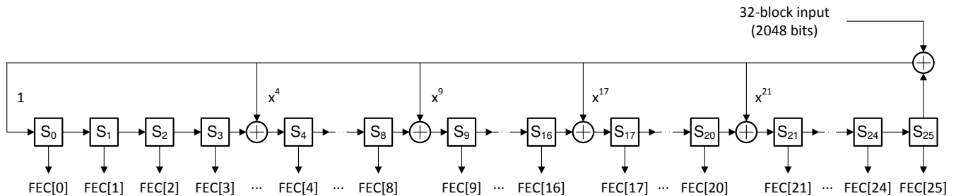
図 6-8. FEC Parity Bit Generator
