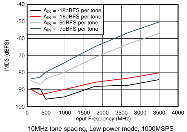
図 5-76. IMD3 vs F_{IN}
