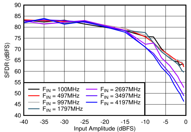
图 5-32. SFDR vs A_{IN}
