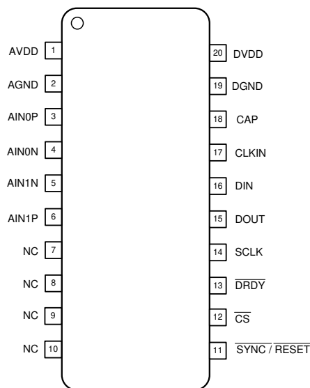
图 5-1. PW Package, 20-Pin TSSOP (Top View)
