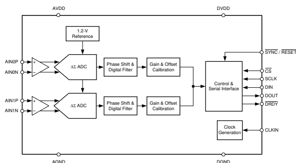
概略ブロック図
