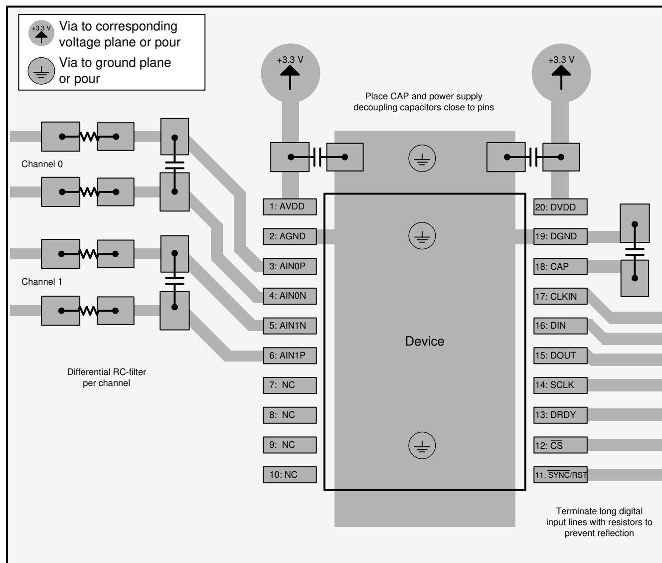
9-6. Layout Example
