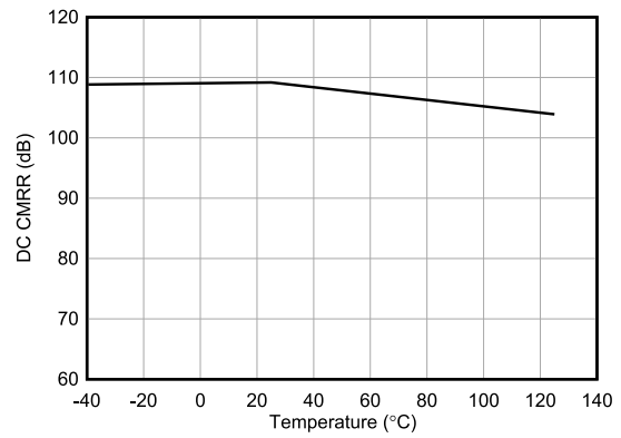
图 6-11. DC CMRR vs Temperature
