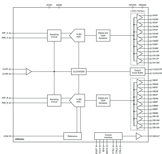
ブロック図
