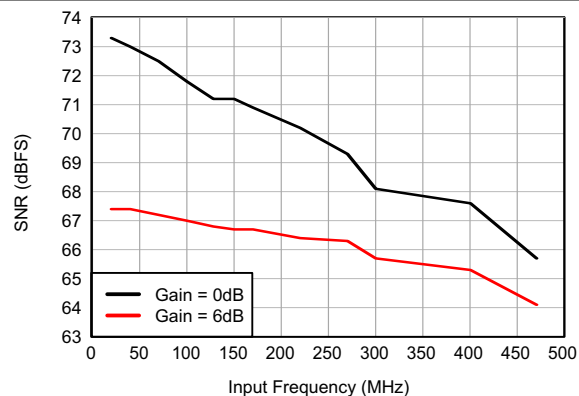
图 6-13. SNR vs Input Frequency (CMOS)
