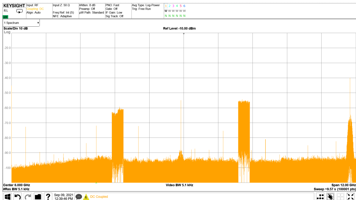
図 4-232. TX 4x100MHz NR Output Spectrum 8.1GHz
