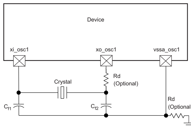
图 6-6. Crystal Implementation
