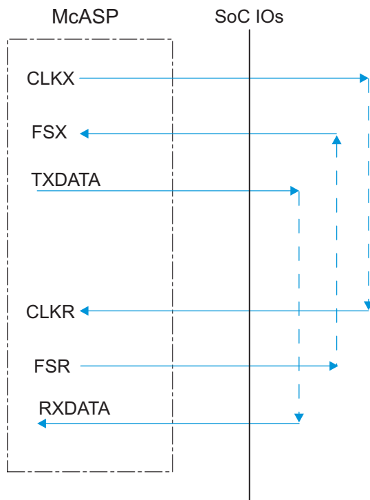
图 7-44. McASP1-8 COFIO - ASYNC Mode
