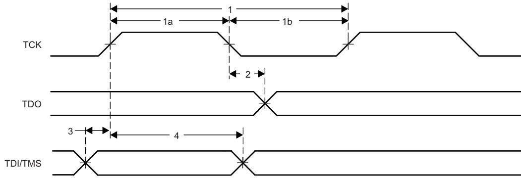
图 7-112. JTAG Timing
