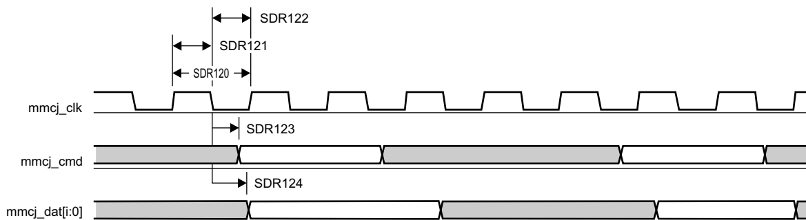
图 7-86. MMC/SD/SDIOj in - SDR12 - Transmitter Mode
