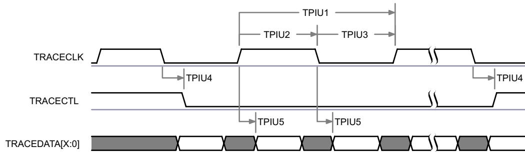
図 7-114. TPIU-PLL DDR Transmit Mode (1)
