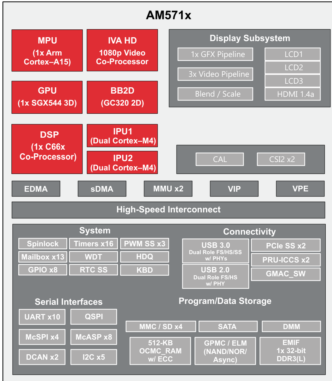
図 1-1. AM571xのブロック図
