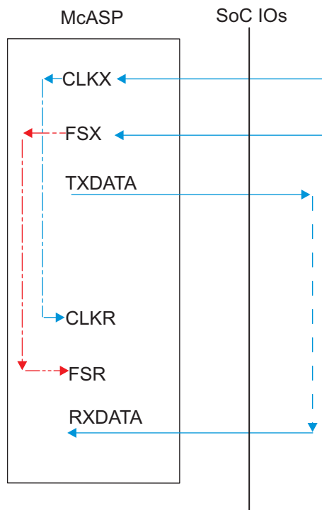
7-49. McASP1-8 CI-FI- - SYNC Mode
