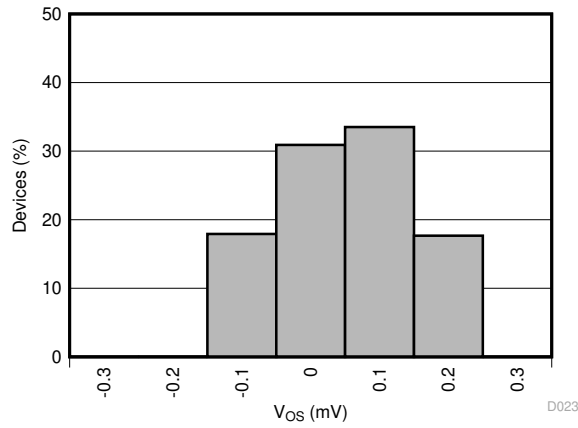
図 5-17. Offset Error Histogram
