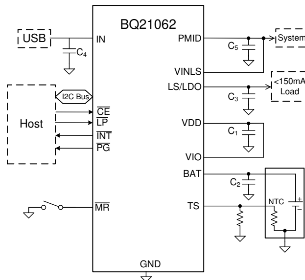
簡略回路図
