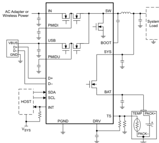
アプリケーション回路図
