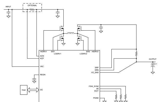
概略回路図
