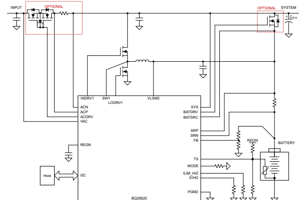
BQ25820 の概略回路図
