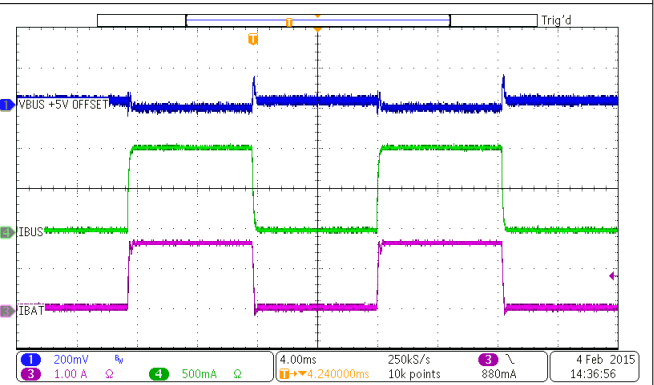
10-9. PFM Switching Waveform
