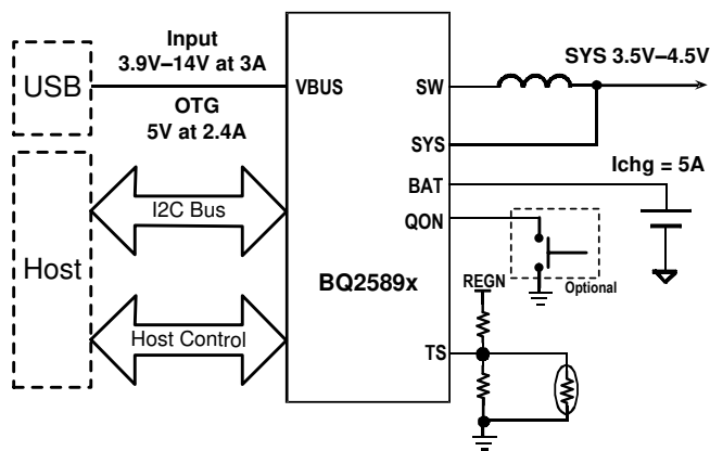
概略回路図
