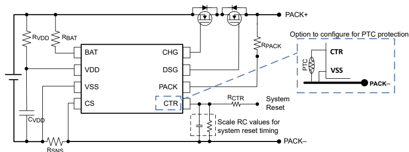
概略回路図
