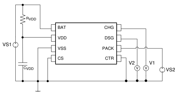
図 8-2. Test Circuit 2
